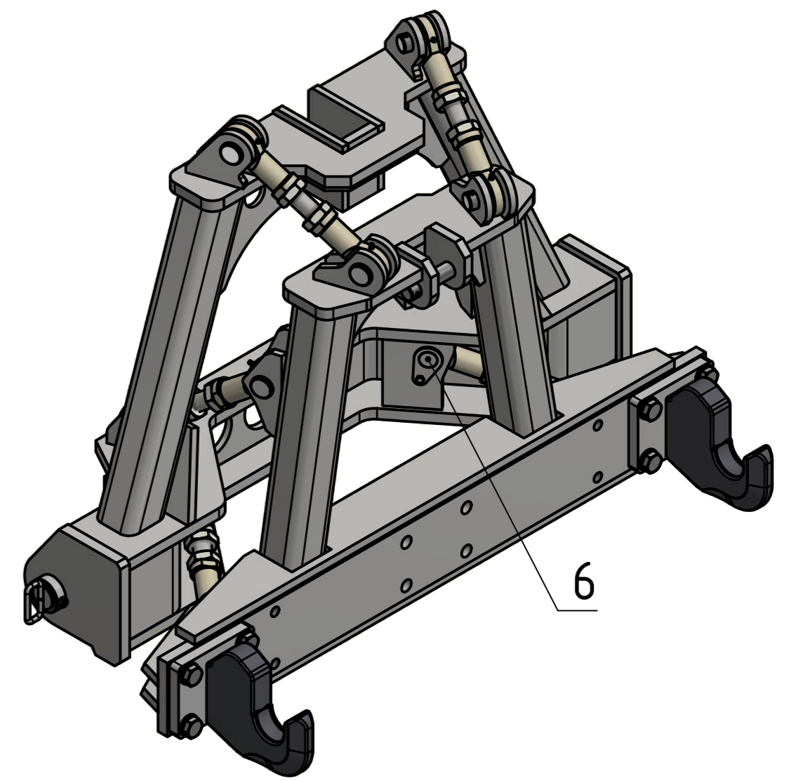
ROZTEČ HÁKŮ NASTAVENA DLE ROZMĚRŮ PRO KATEGORII 4
