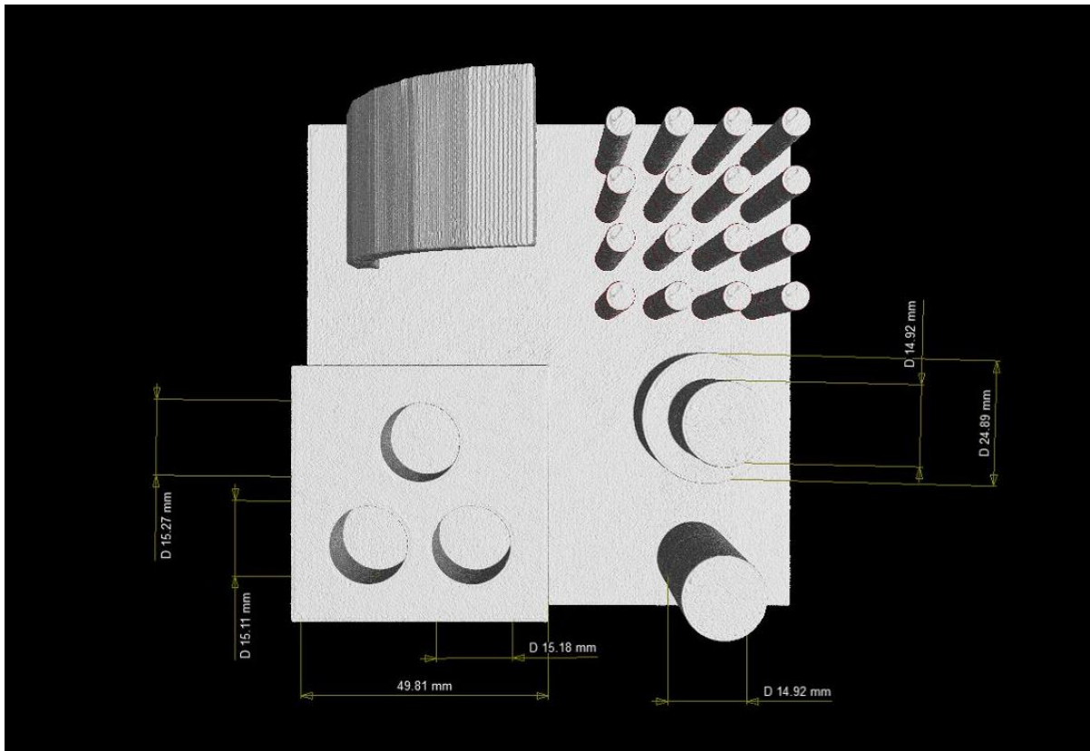
Obr. 6 Rozměry Verbatim
