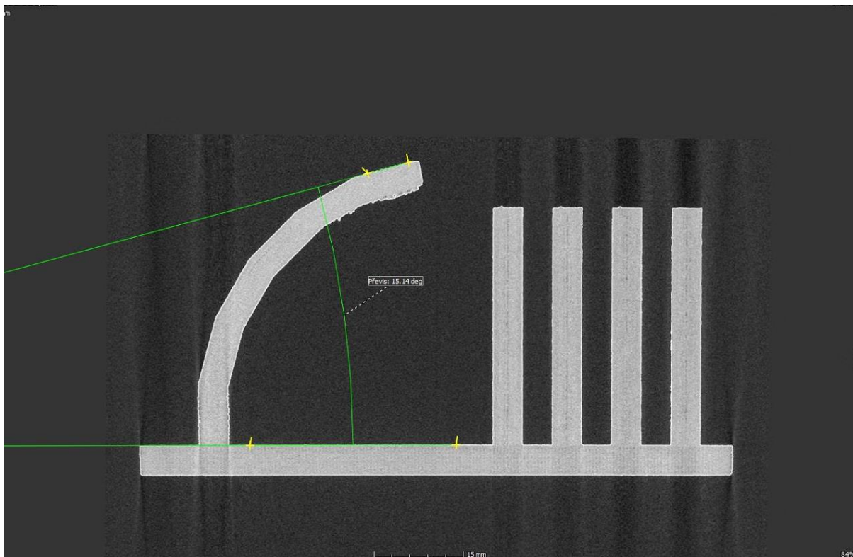
Obr. 5 Úhel převisu Prusament
