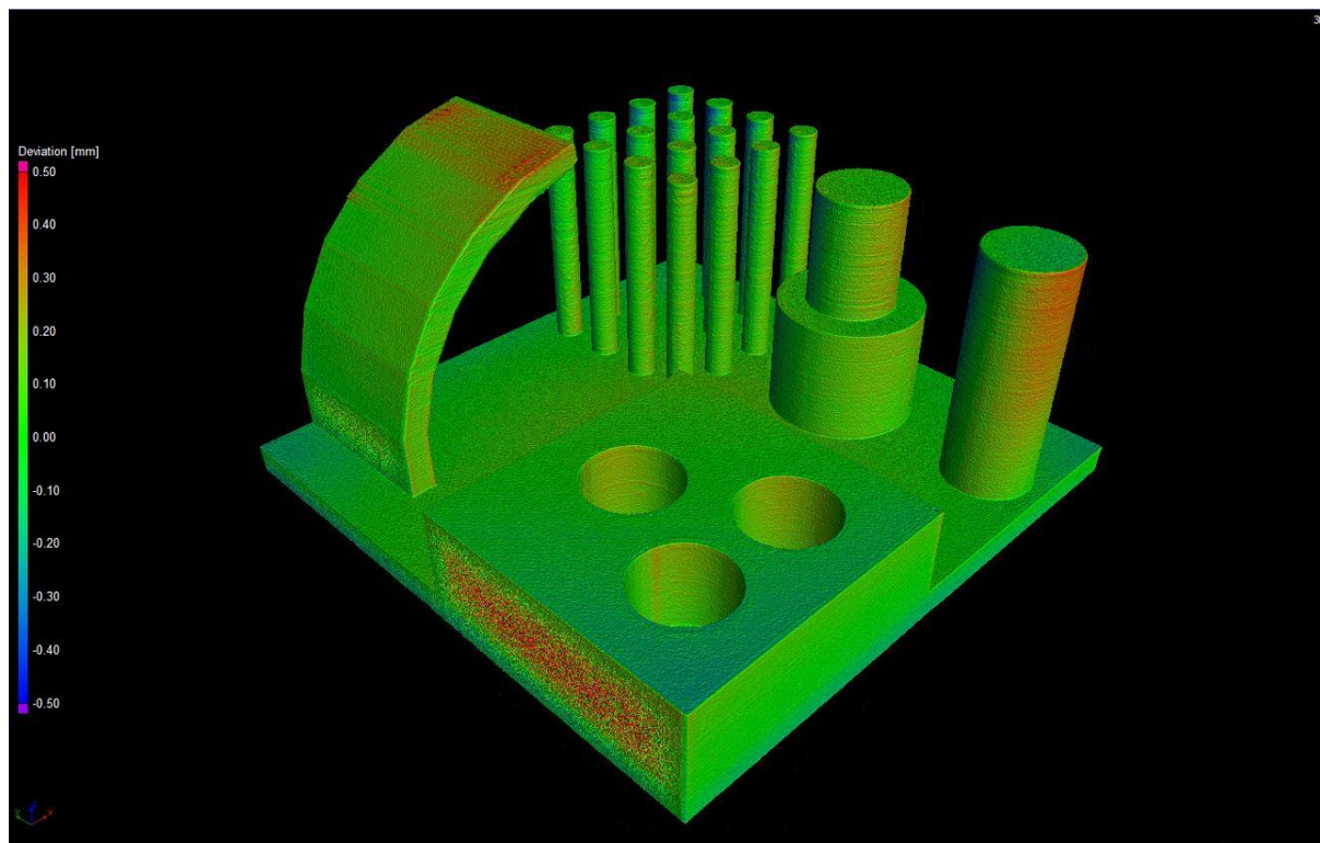
Obr. 1 Barevná mapa Prusament
