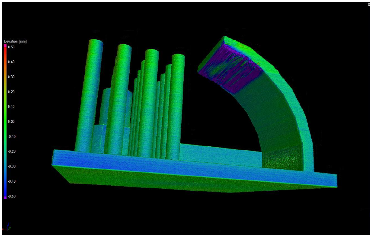
Obr. 3 Převis detail Prusament
