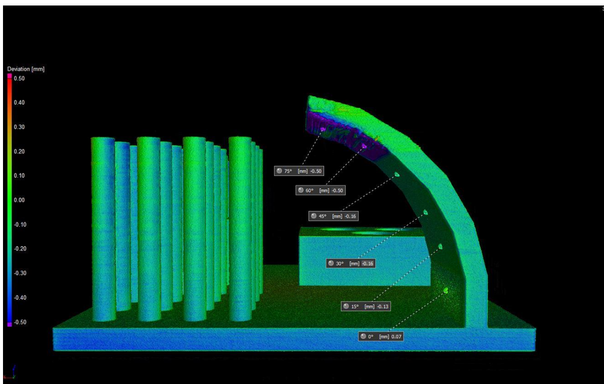
Obr. 4 Převis odchylky Prusament
