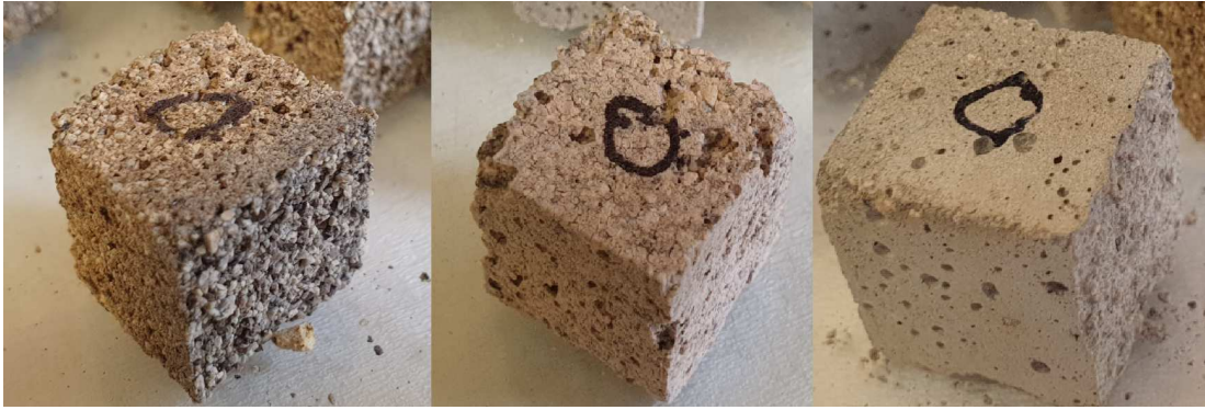
Obrázek 10 - Vzorky malt, kostky, výpal 900 °C 6A,6B,6C
