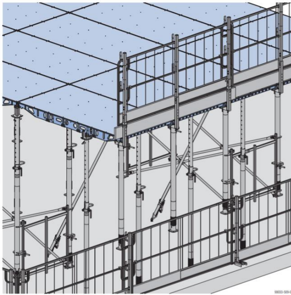
Bednění stropu
