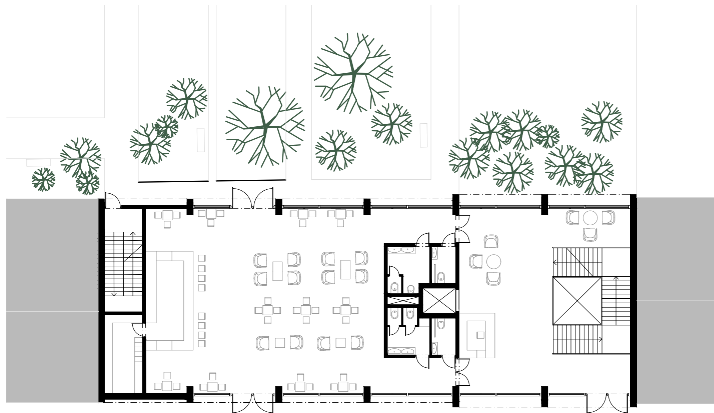
RŮŽOVÁ 1NP
