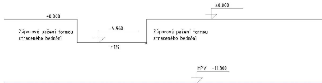
Schematický příčný řez stavební jámou
