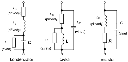
Obr. 7 Schémata náhradních obvodů základních pasivních součástek.
