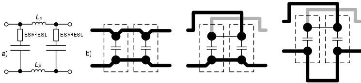
Obr. 9 Dvojice paralelně spojených kondenzátorů (a) schéma; (b) plošné spoje pro kompenzaci.
