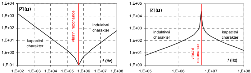
Obr. 8 Absolutní velikost impedance kondenzátoru 1 \mu\text{F} (vlevo) a cívky 10 \mu\text{H} (vpravo).
