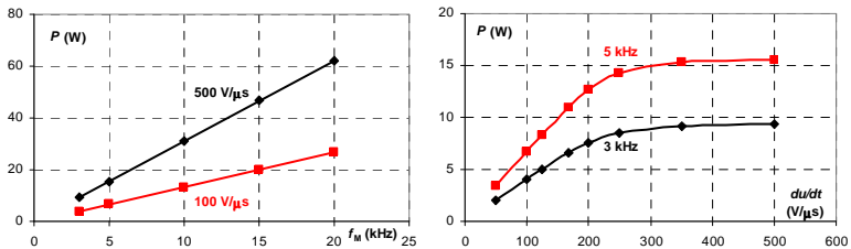
Obr. 24 Vliv modulačního kmitočtu a strmosti výstupního napětí na ztráty.
