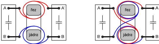
Obr. 13 Půdorys možného uspořádání filtru. Standardní propojení (vlevo) a plně symetrické (vpravo) vinutí kompenzovaných cívek vzhledem k dvojici kapacit.
