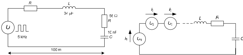
Obr. 22 Zjednodušený obvod pro výpočet ztrát v sinusovém, du/dt filtru a terminátoru.
