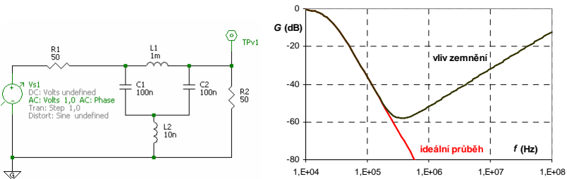
Obr. 6 Vliv zemničícího vodiče na nesymetrický přenos (simulace v 5Spice Analysis).
