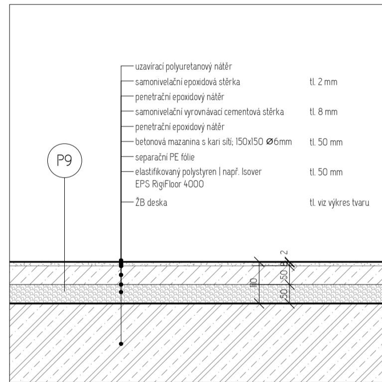
Sklad
