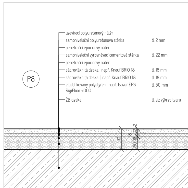
Kancelář, šatna
