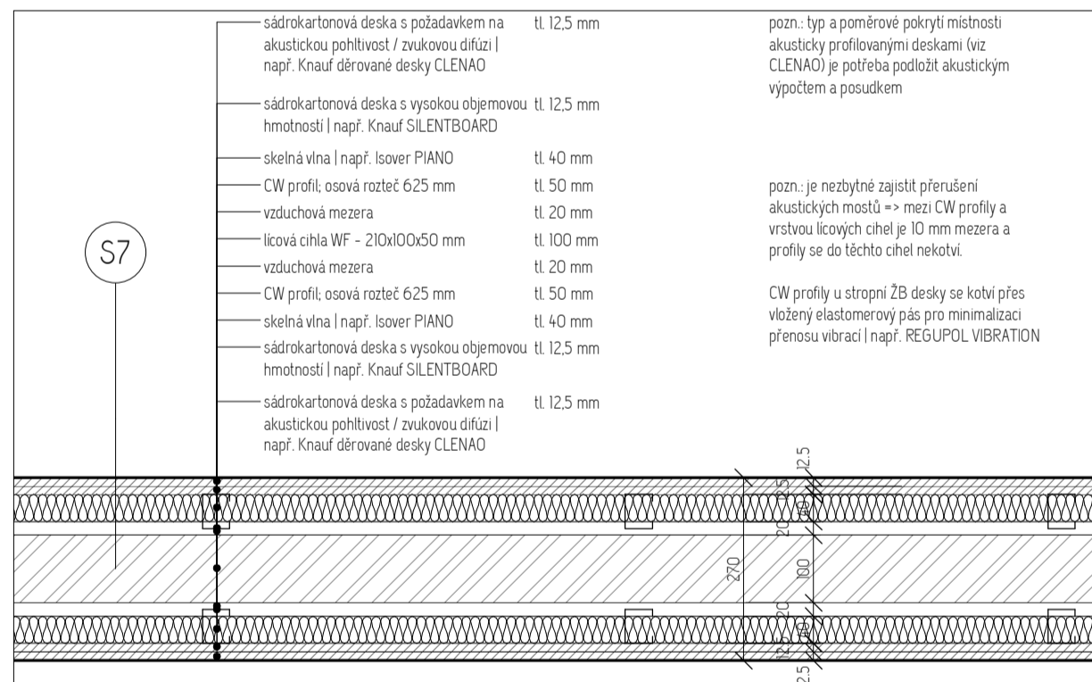
Hudební učebny
