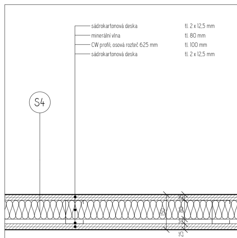
Kanceláře, šatny
