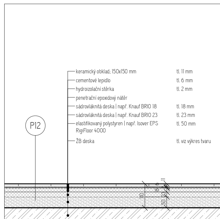
WC, umývárna
