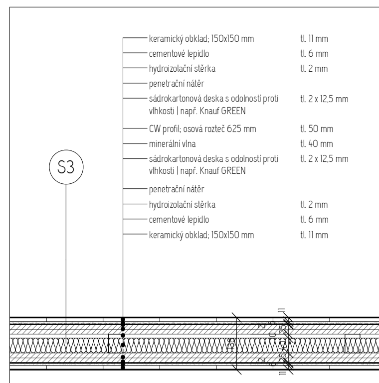
WC, koupelny
