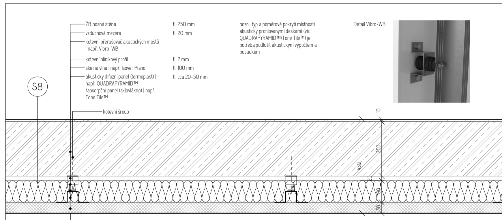
Koncertní sál
