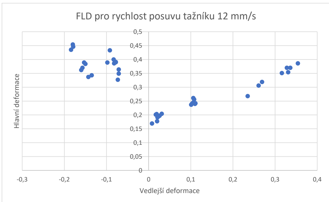
Obr. 2, FLD pro rychlost posuvu tažníku 12 mm/s
