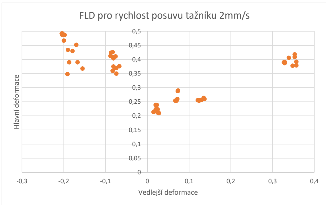
Obr. 1, FLD pro rychlost posuvu tažníku 2 mm/s
