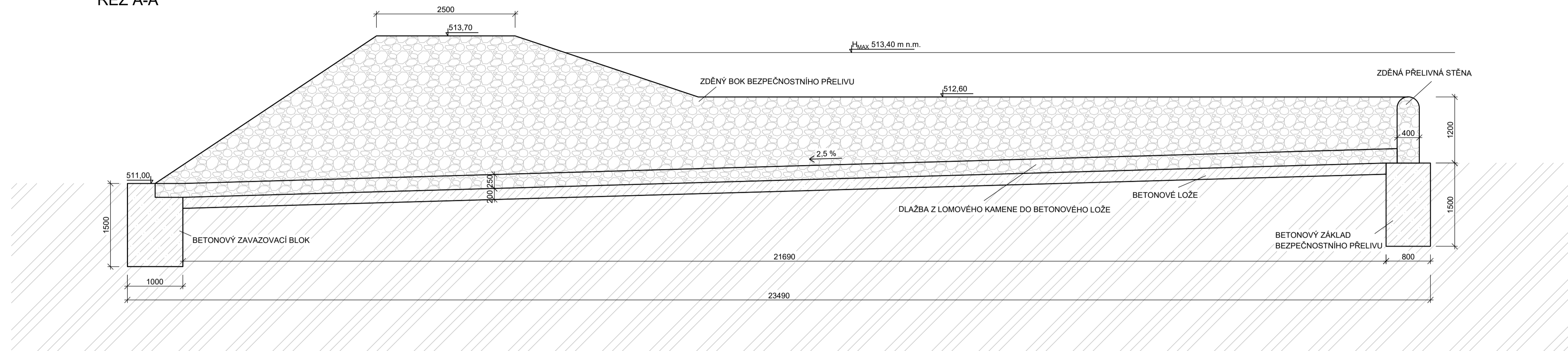
ŘEZ A-A'
