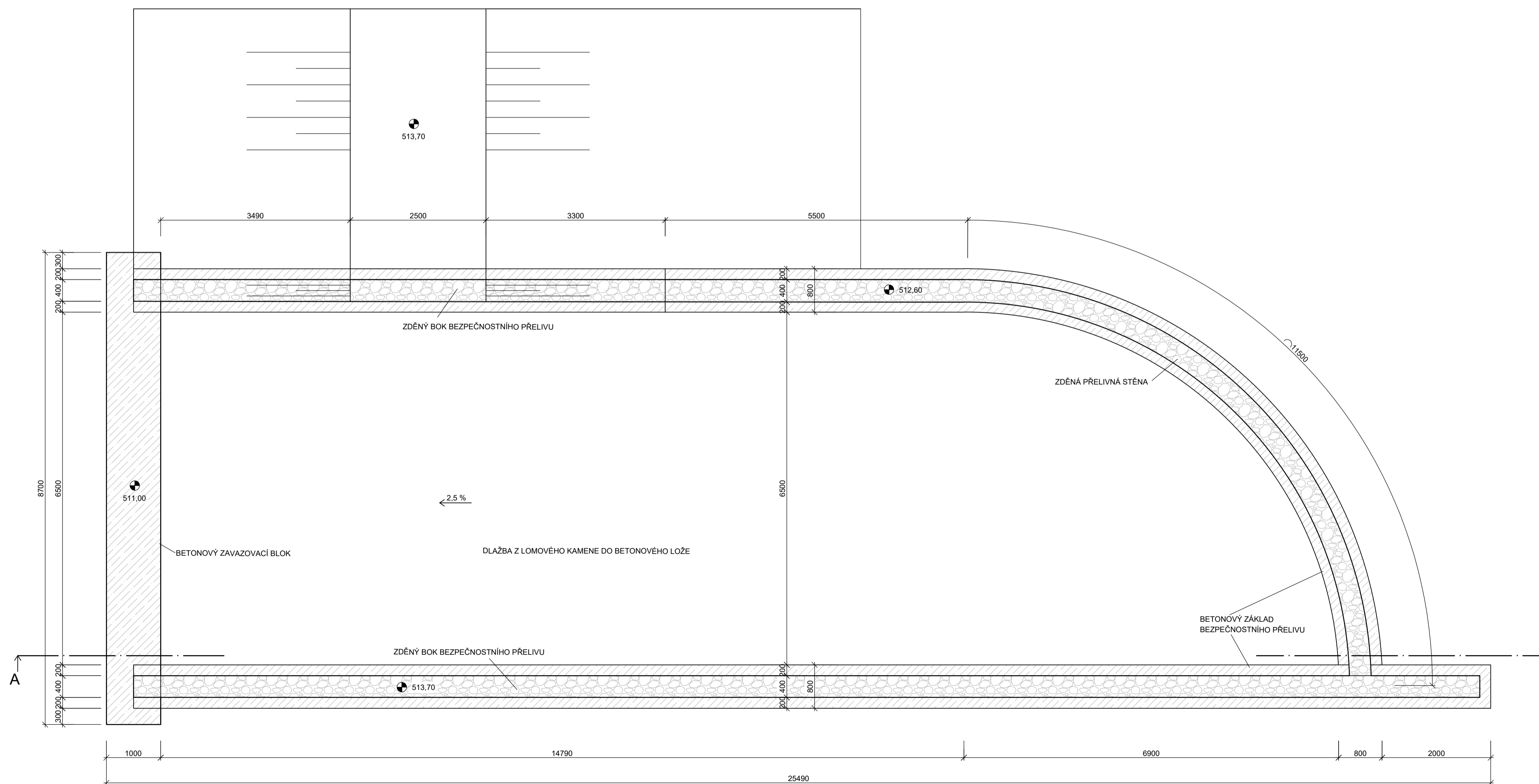
PŮDORYS
