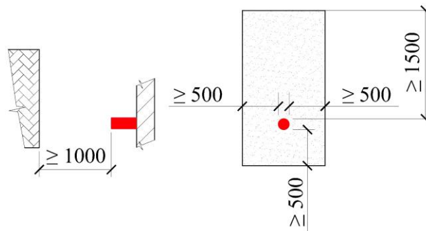
Obr. 6 Předepsané minimální odstupné vzdálenosti pro umístování hořlavých materiálů od horizontálního vyústění spalin na venkovní zdi
