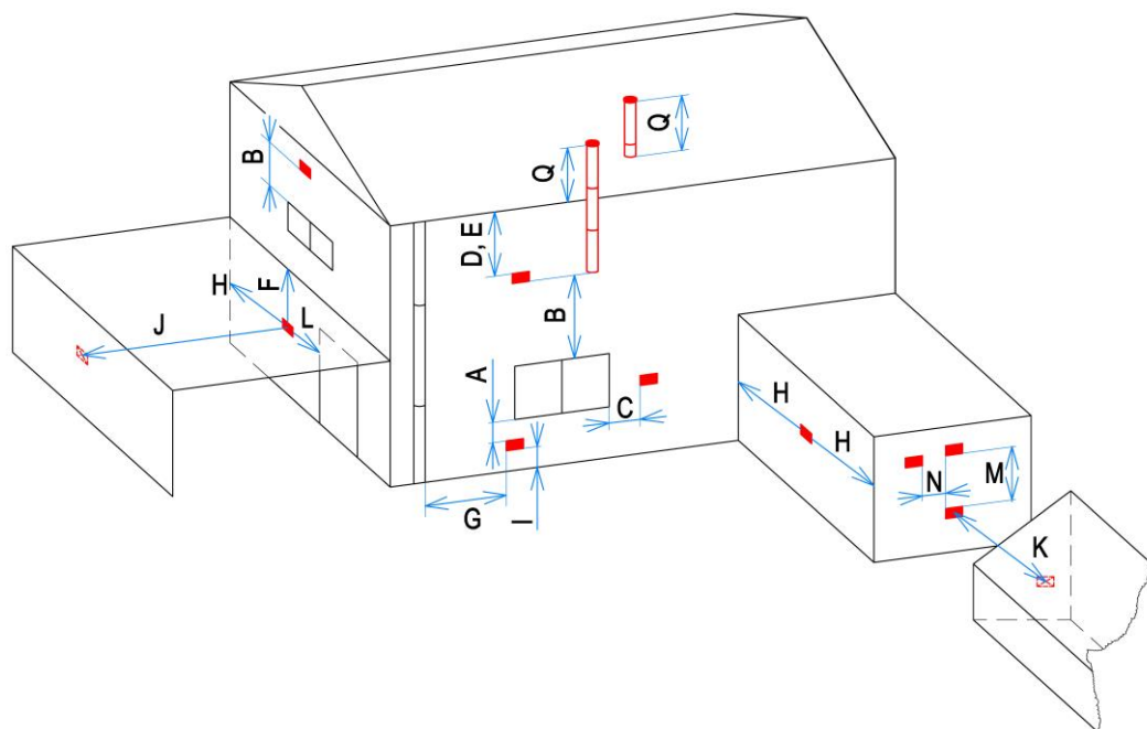
Obr. 1 Příklady polohy vyústění vyvážených komínových soustav (ČSN EN 15287-2) [L2]
