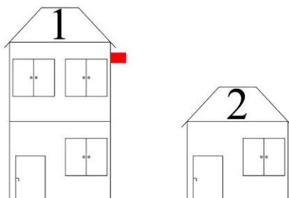
Obr. 3 Příklad vyústění odtahu spalin venkovní stěnou budovy 1 nad úroveň budovy 2 - vzdálenost mezi budovami se neposuzuje. Budova 1 se považuje a samostatně stojící budovu
