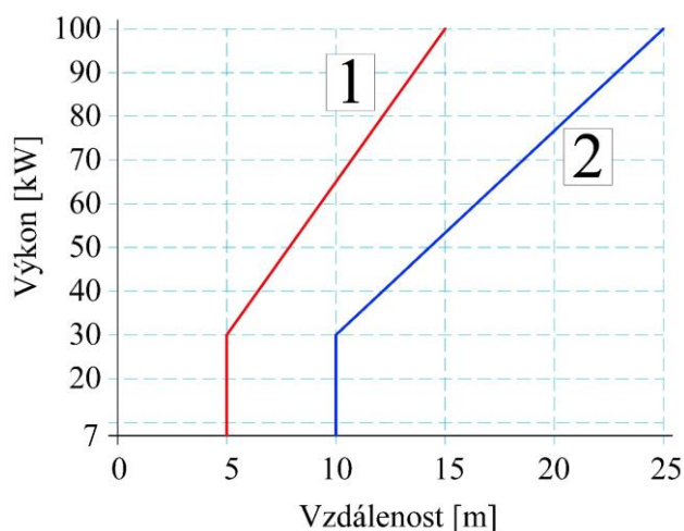
Obr. 8 Předepsané vzdálenosti sousedních nebo protilehlých budov odtahu spalin u průmyslových budov
