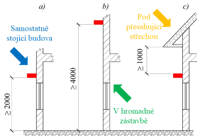
Obr. 5 Předepsané vzdálenosti vyústění spodní hrany kouřovodu na obvodové zdi nad okolním terénem
