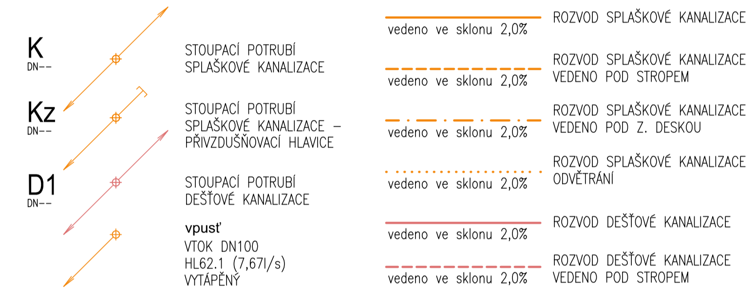
LEGENDA KANALIZACE:
