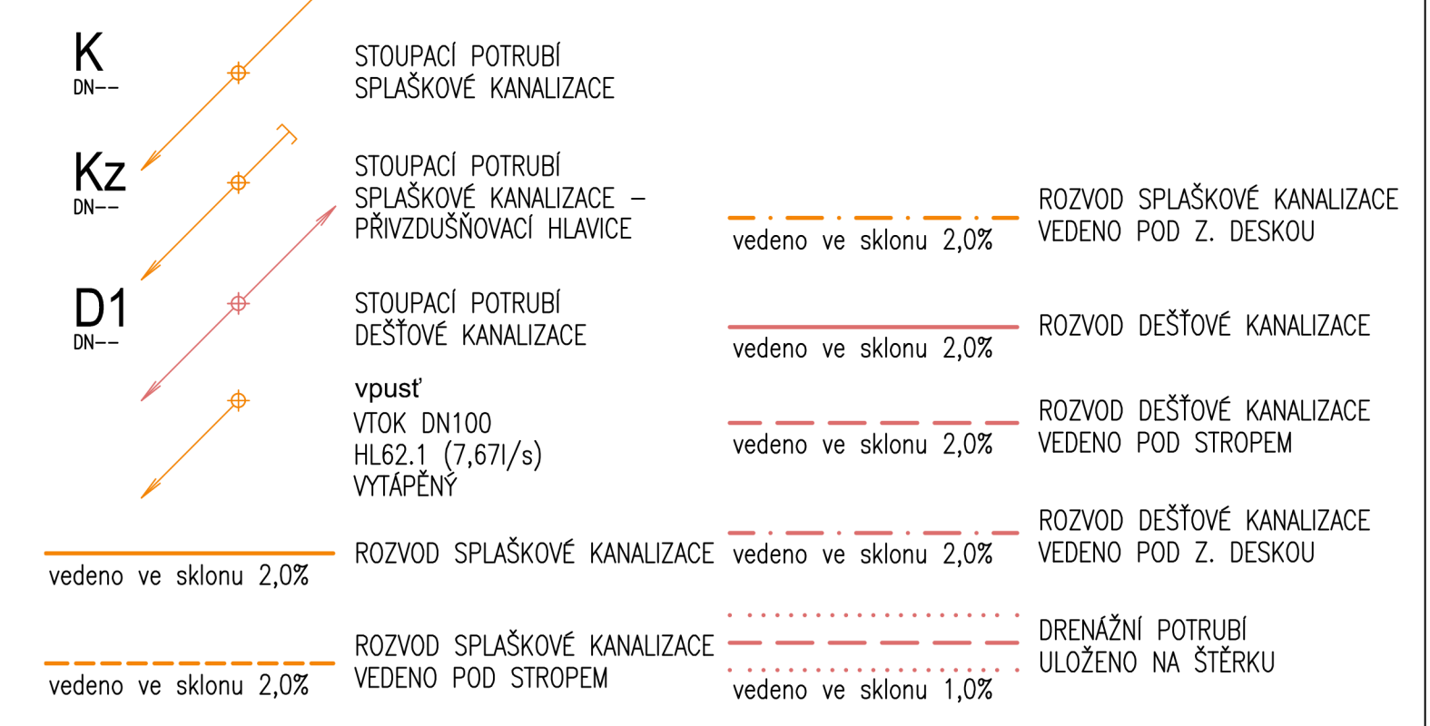
LEGENDA KANALIZACE:
