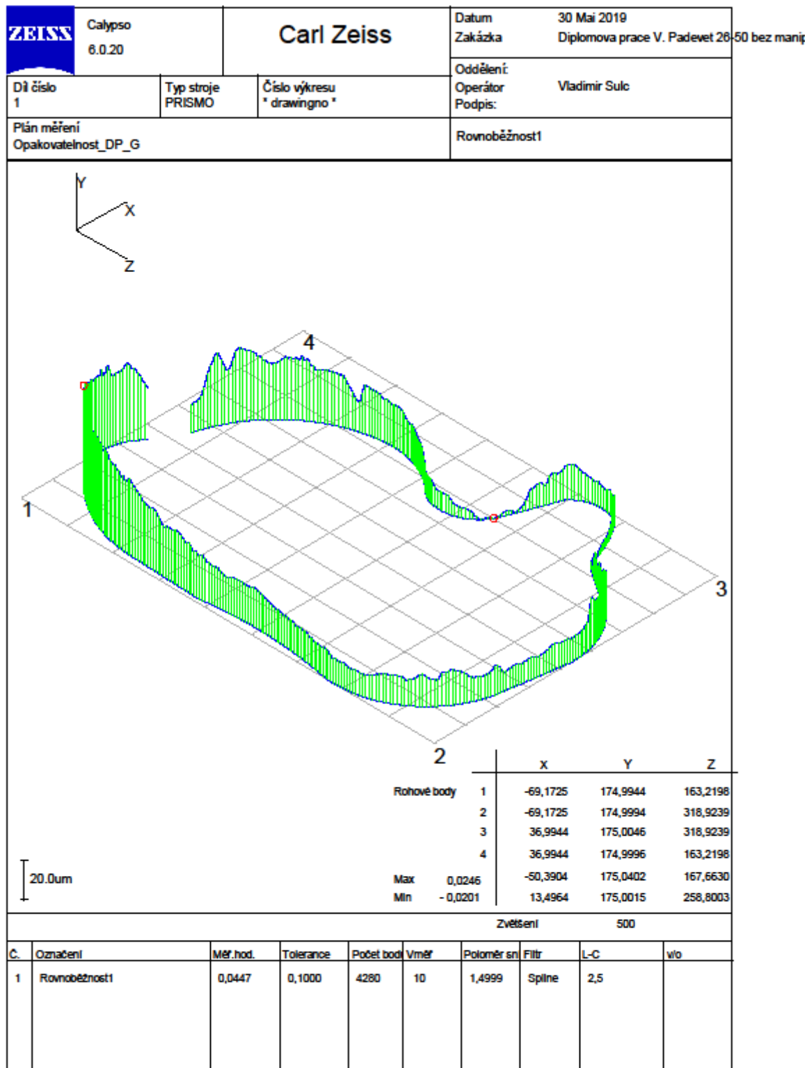
Příloha 3: Profil roviny 3 pro maximální hodnotu rovnoběžnosti
