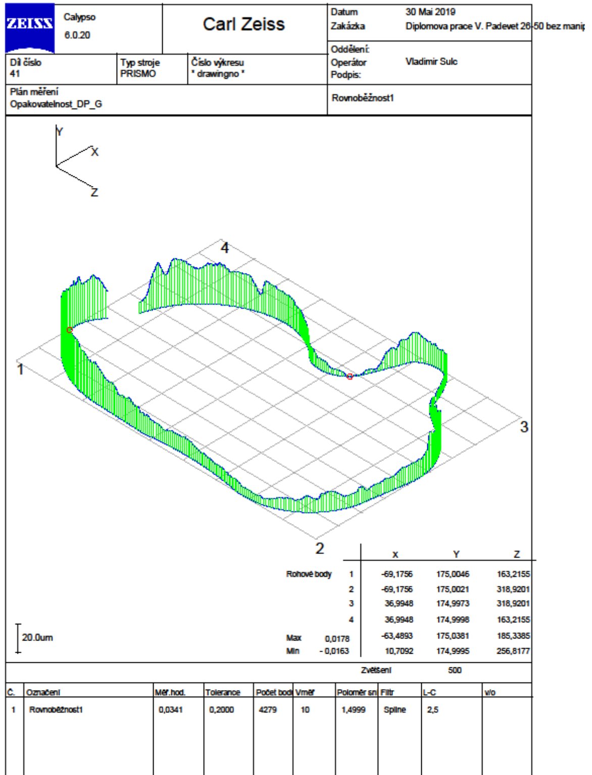
Příloha 5: Profil roviny 3 pro minimální hodnotu rovnoběžnosti
