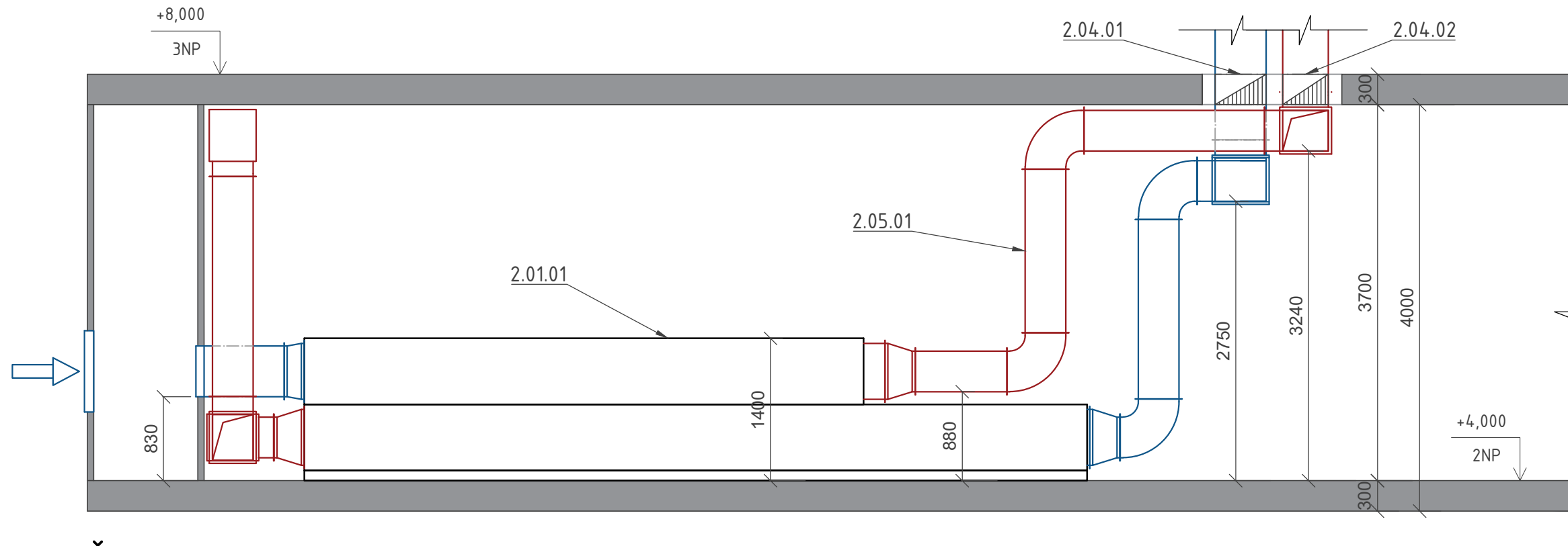
ŘEZ A
