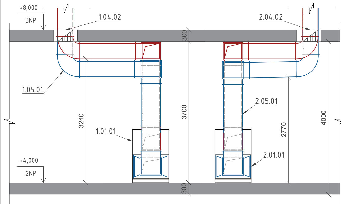
ŘEZ B
