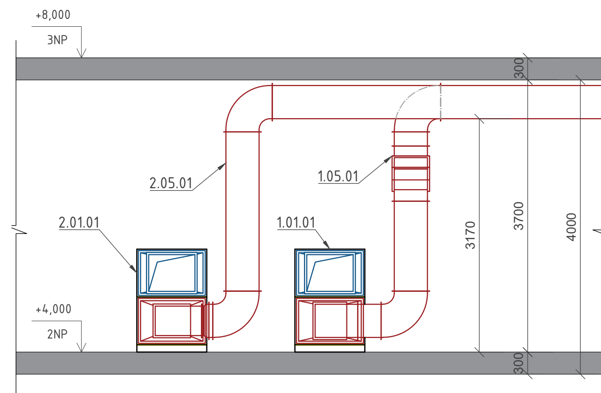
ŘEZ C
