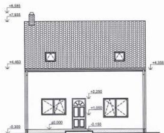
POHLED SEVERNÍ
