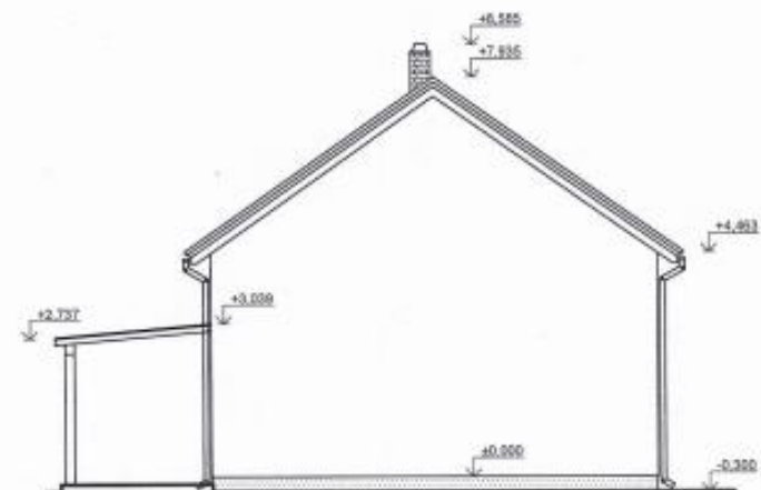
POHLED ZÁPADNÍ
