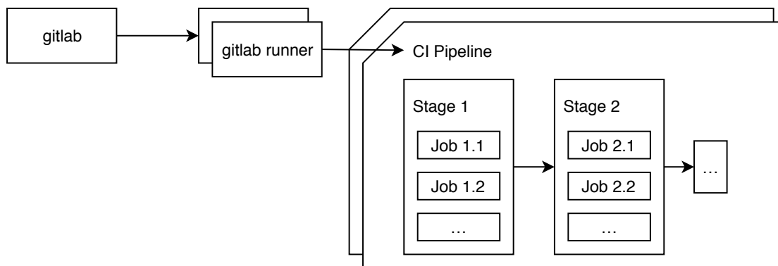
Fig. 2.5: Architektura GitLab CI. Runnerů i pipeline může existovat mnoho. V rámci jedné pipeline je několik stages, uvnitř kterých je sada paralelně spuštěných jobs.
