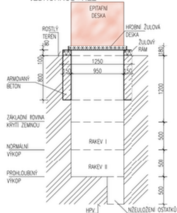
Obrázek č. 27 - Náčrt jednohrobu a dvouhrobu
