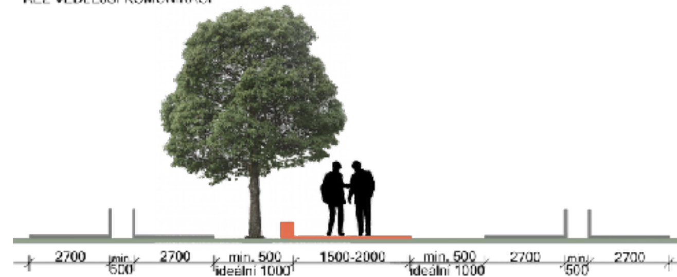
Obrázek č. 21 - Řez vedlejší komunikací - vzorový příklad
