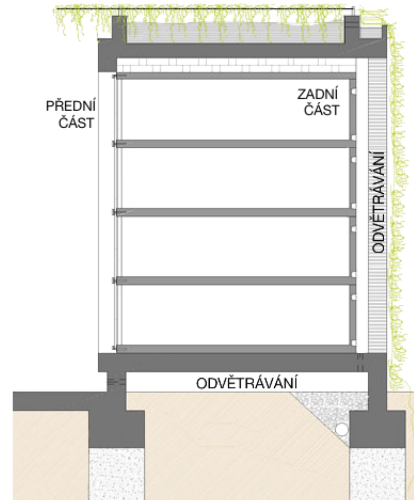
Obrázek č. 2 -Řez hrobu typu „nicho“
