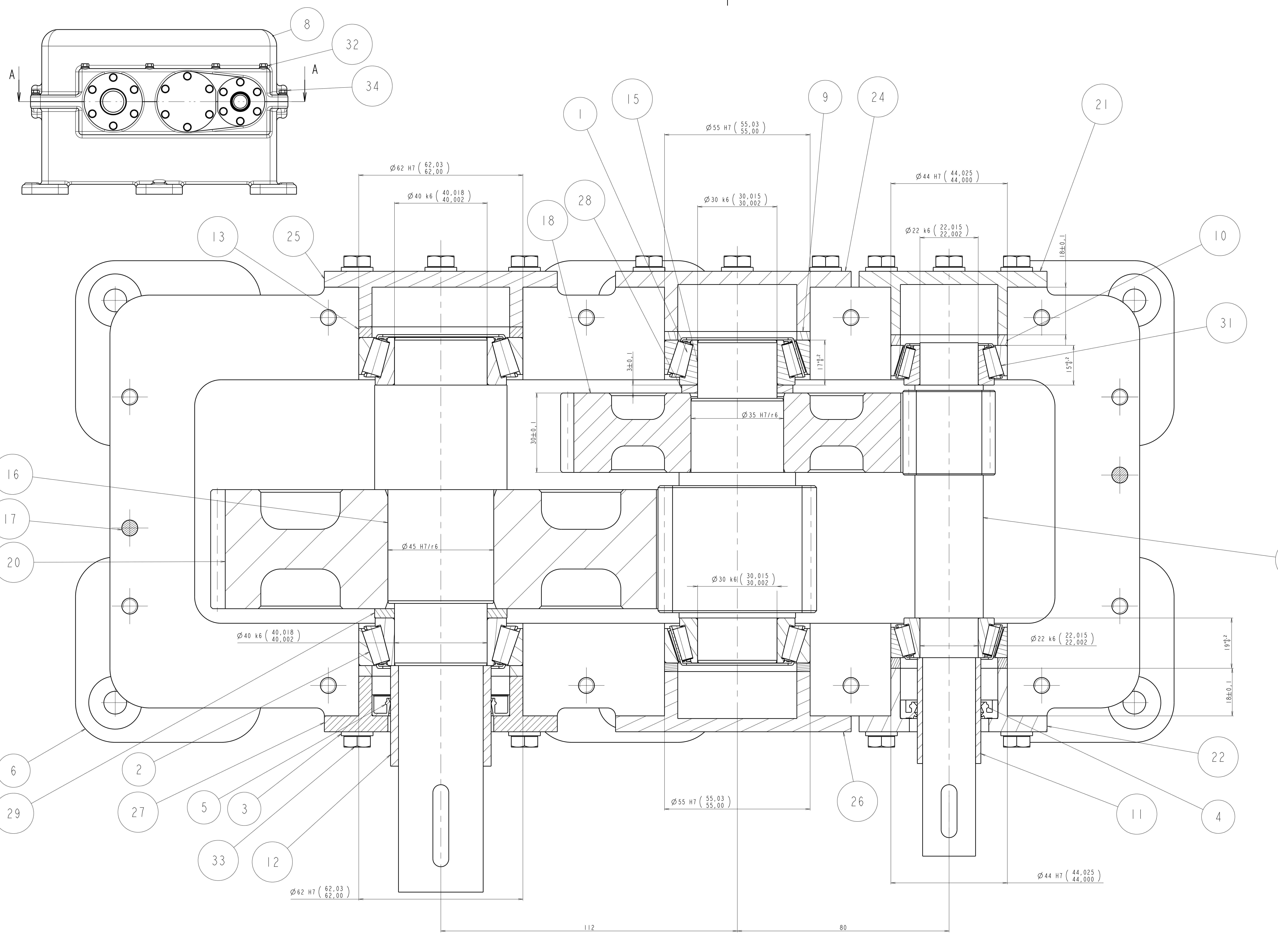
A - A 2:1
