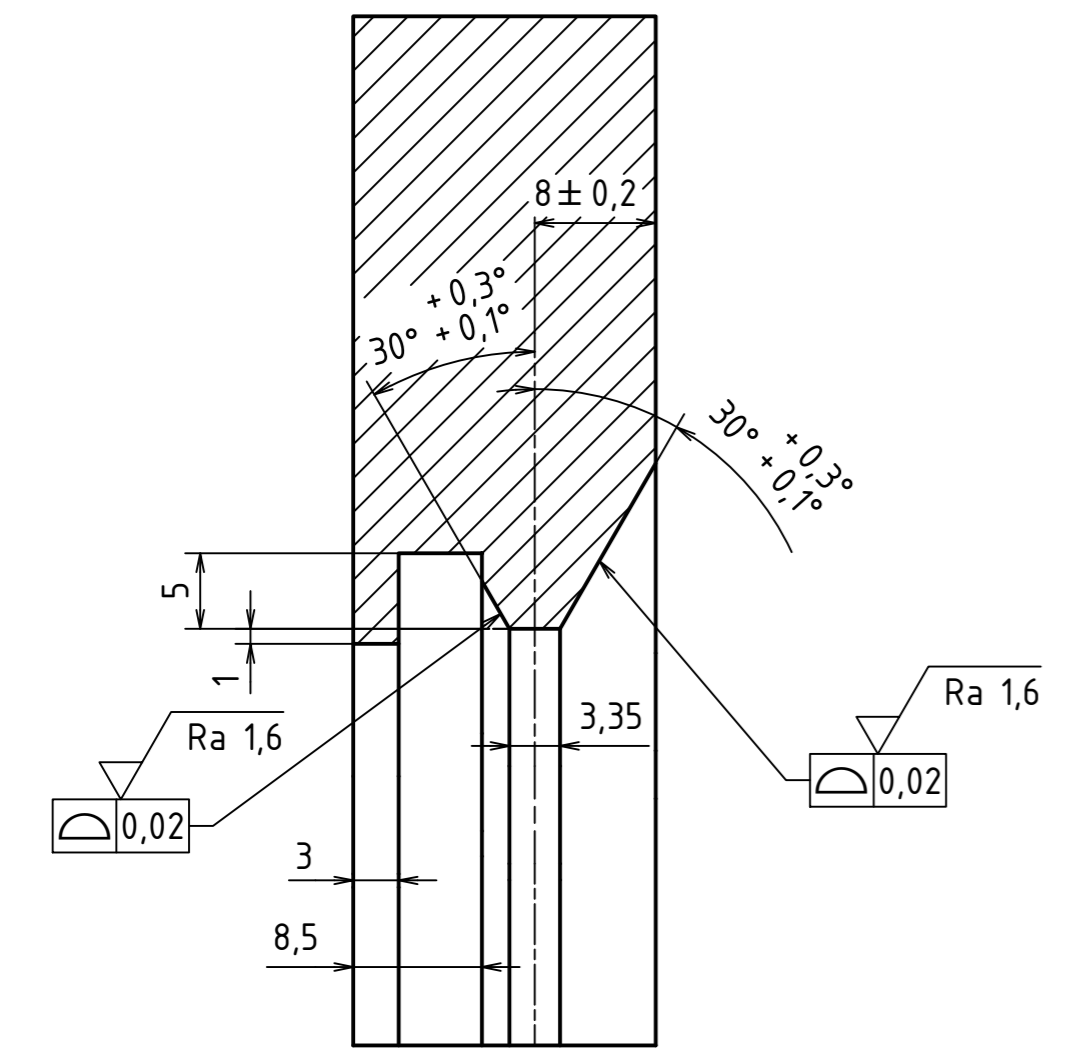
B-B 2 : 1
