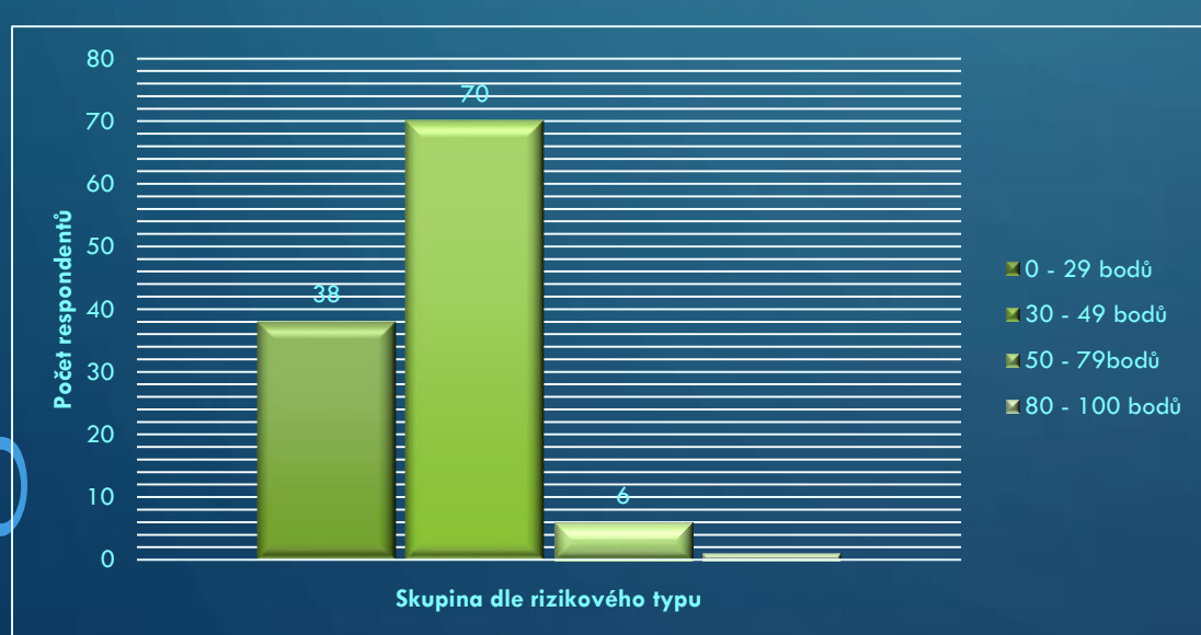
Histogram výsledků testu dle Kimberly Young
