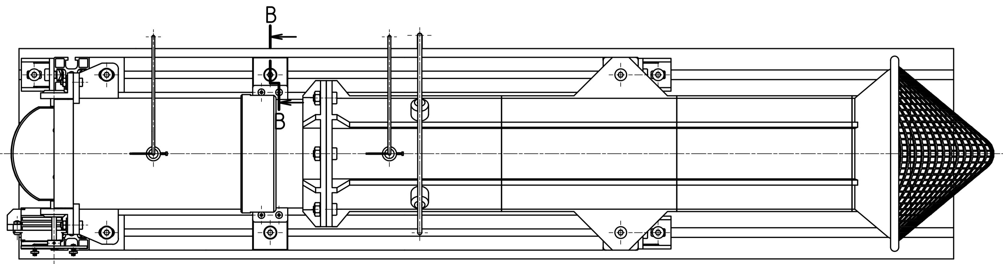
PŮDORYS ZOBRAZEN BEZ OCHRANNÝCH KRYTŮ PRO VIDITELNOST UCHYCENÍ SESTAVY DMYCHADLA
