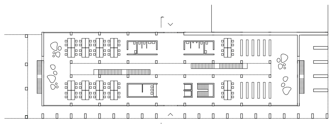
1. nadzemné podlažie
