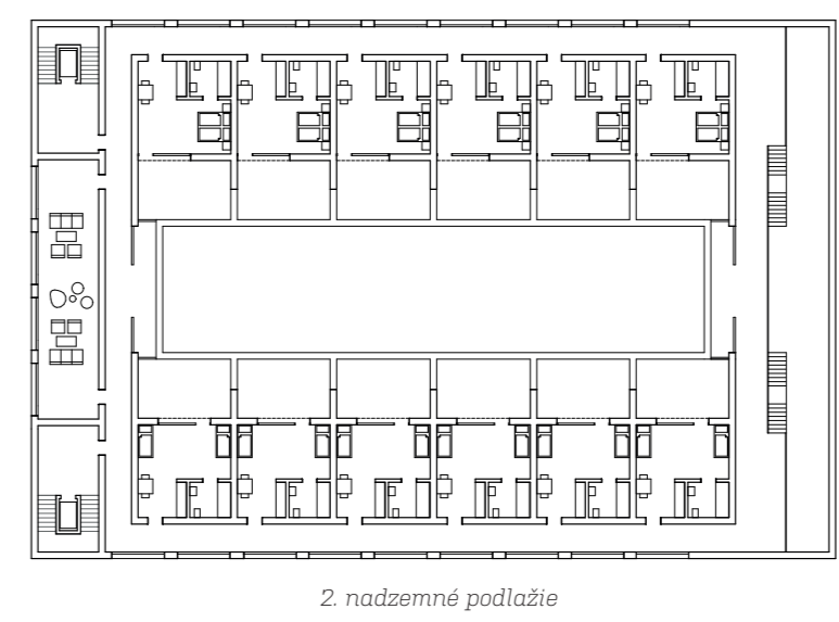
2. nadzemné podlažie
