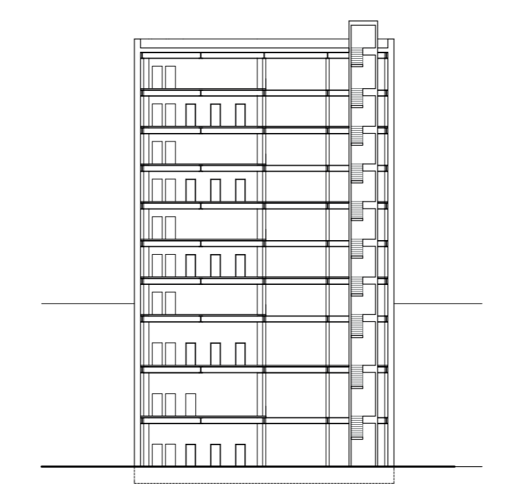
rez balkónmi
