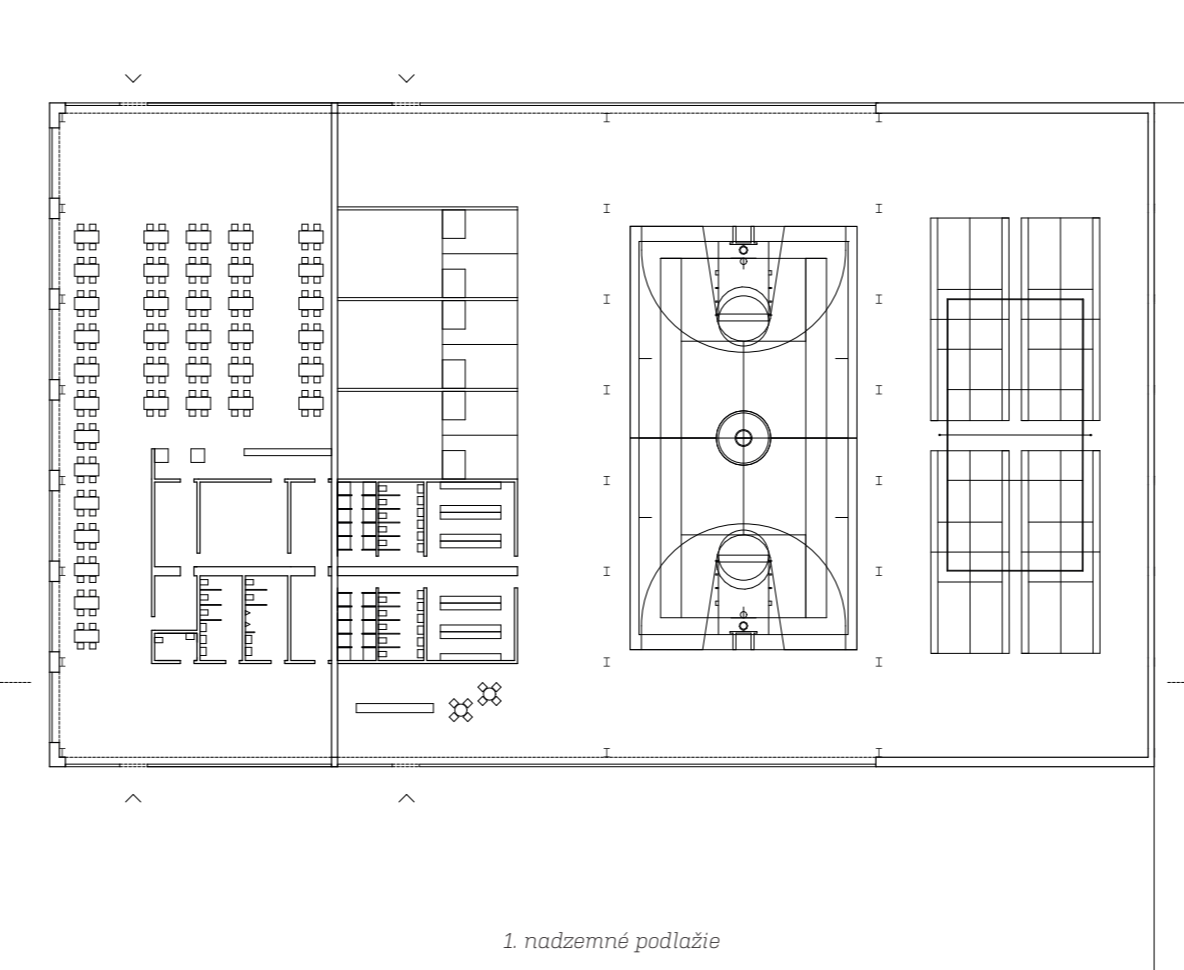
1. nadzemné podlažie
