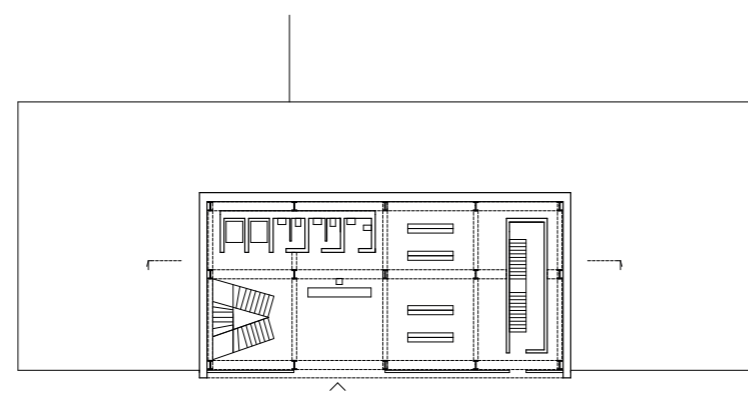
1. nadzemné podlažie
