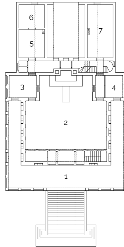
první patro
