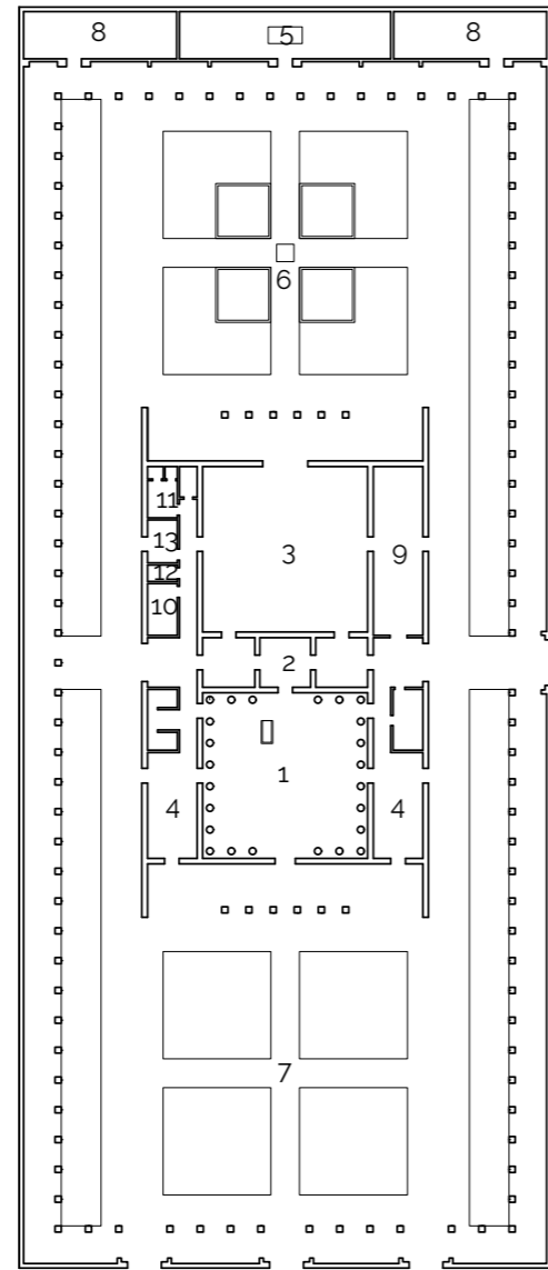
přízemí
