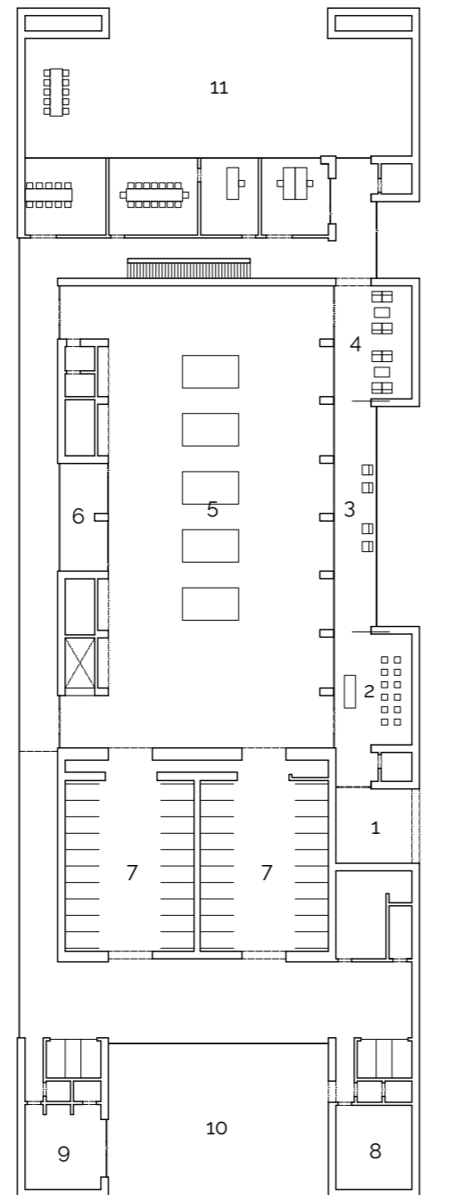
přízemí
