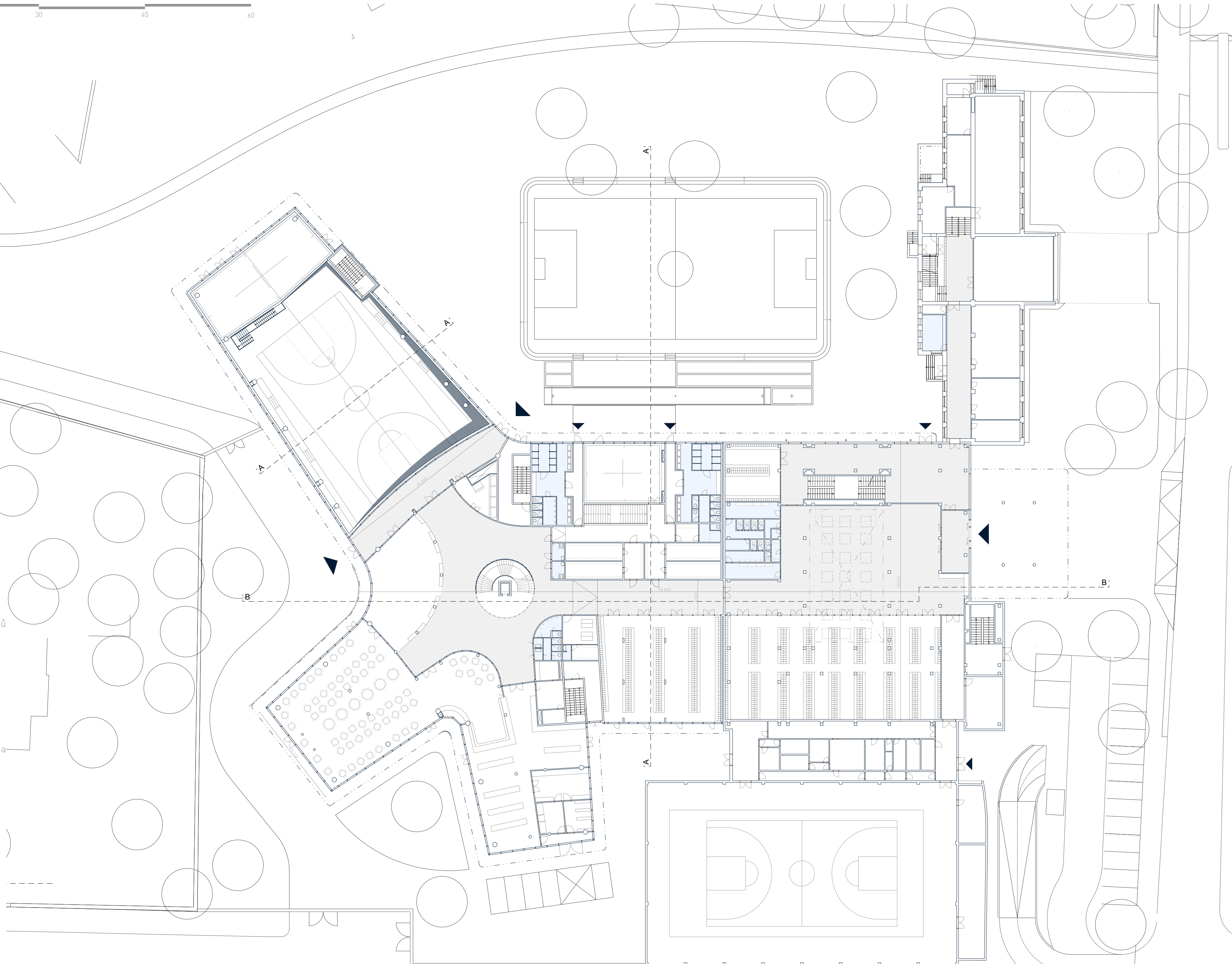
Půdorys přízemí
