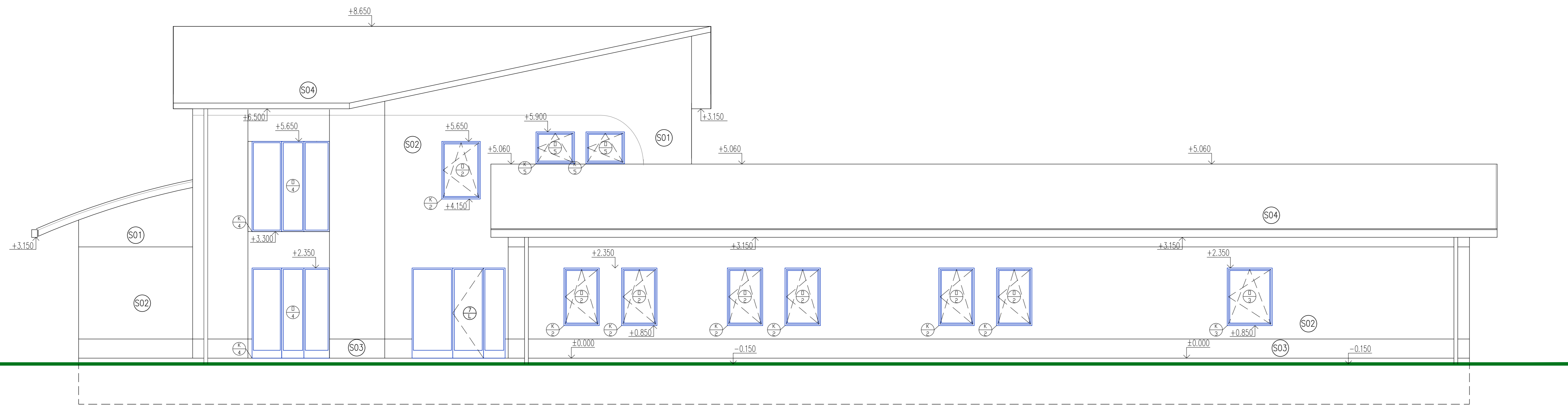
POHLED VÝCHODNÍ
