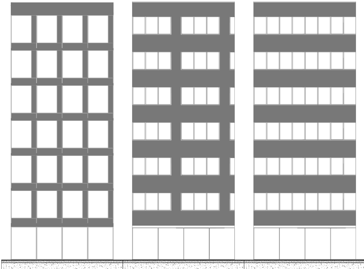
PŮVODNÍ FASÁDA
