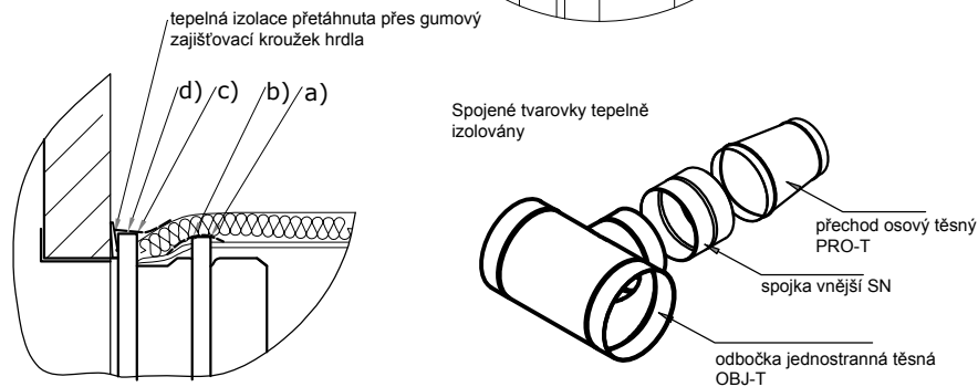
Detail 2: HRDLO JEDNOTKY + SONOFLEX
