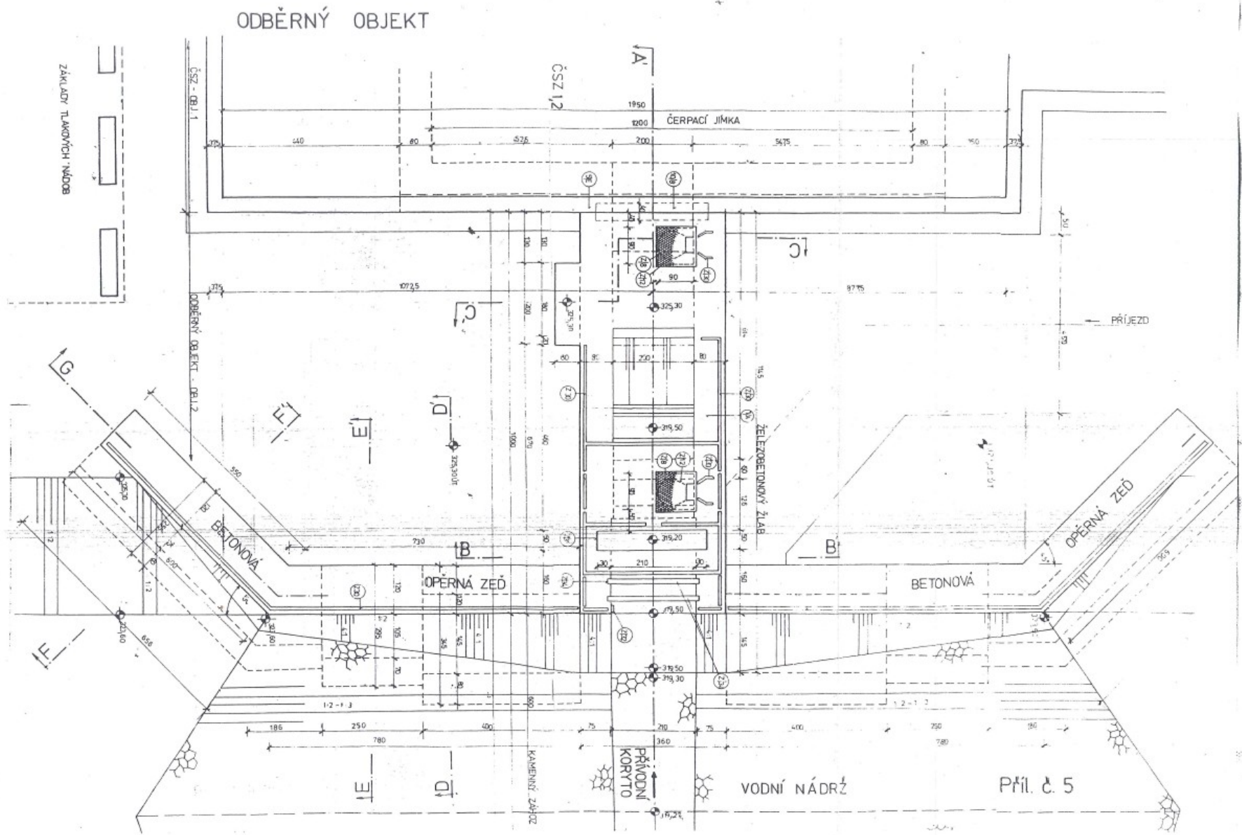
Příloha C: Situace odběrného objektu [2]
