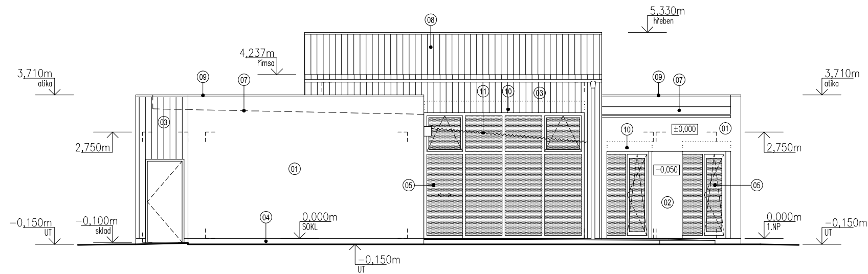
POHLED SEVEROZÁPADNÍ
