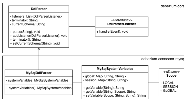
Obr. 6.1: Diagram tried aktuálneho návrhu MySQL DDL parseru
