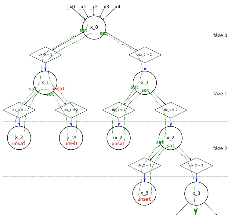
Obrázek 3.2: Ilustrace postupu základního algoritmu prohledávaným prostorem
