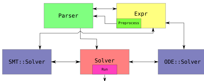
Obrázek 4.1: Blokové schéma modelu komponent implementovaného prototypu
