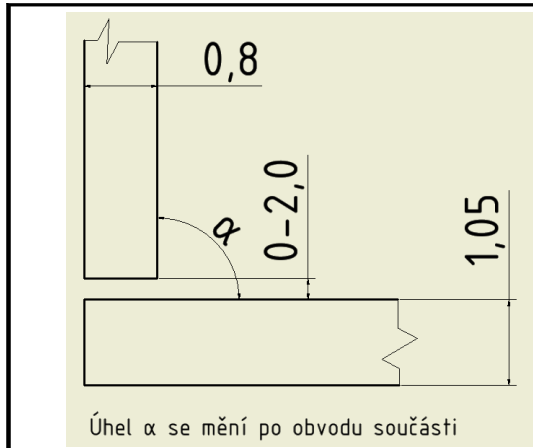
Návrh spoje
