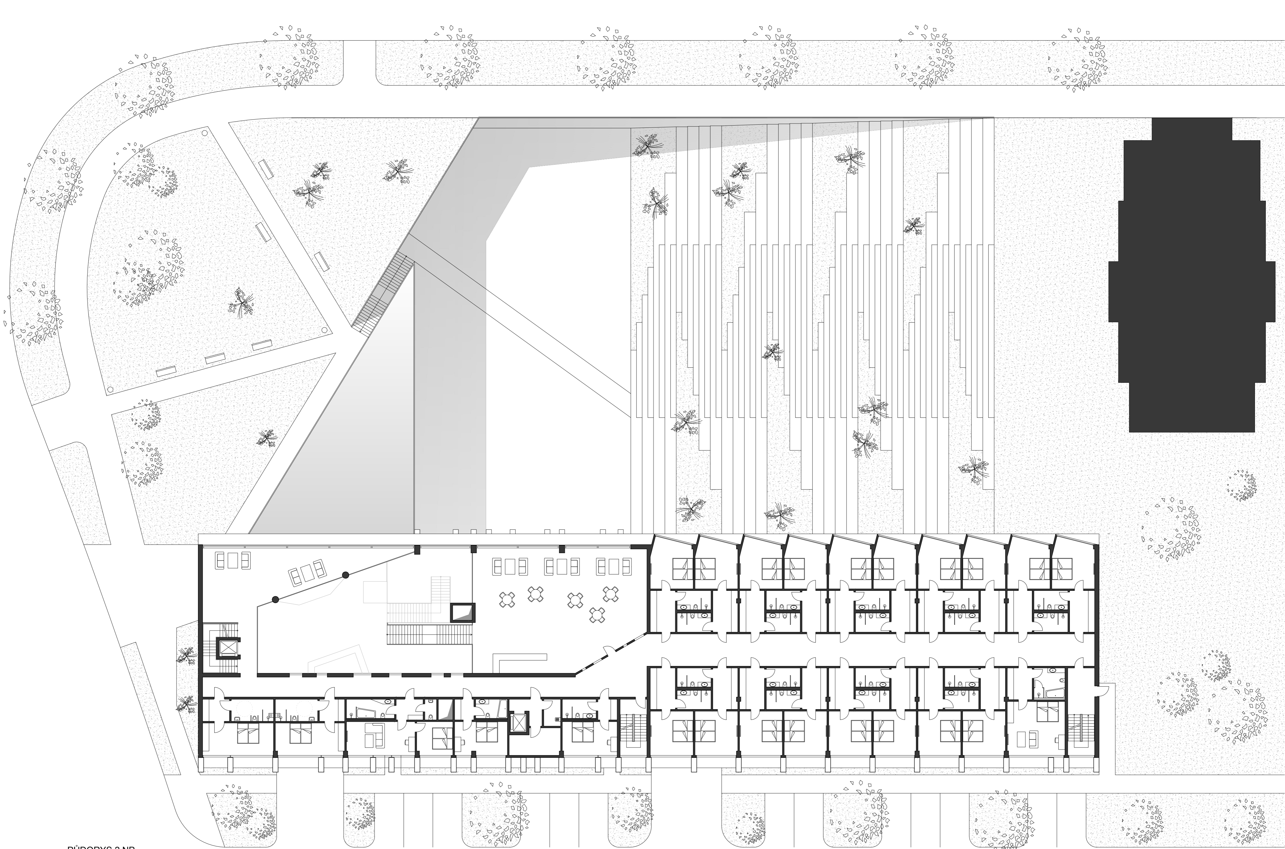
PŪDORYS 2.NP 1:200
