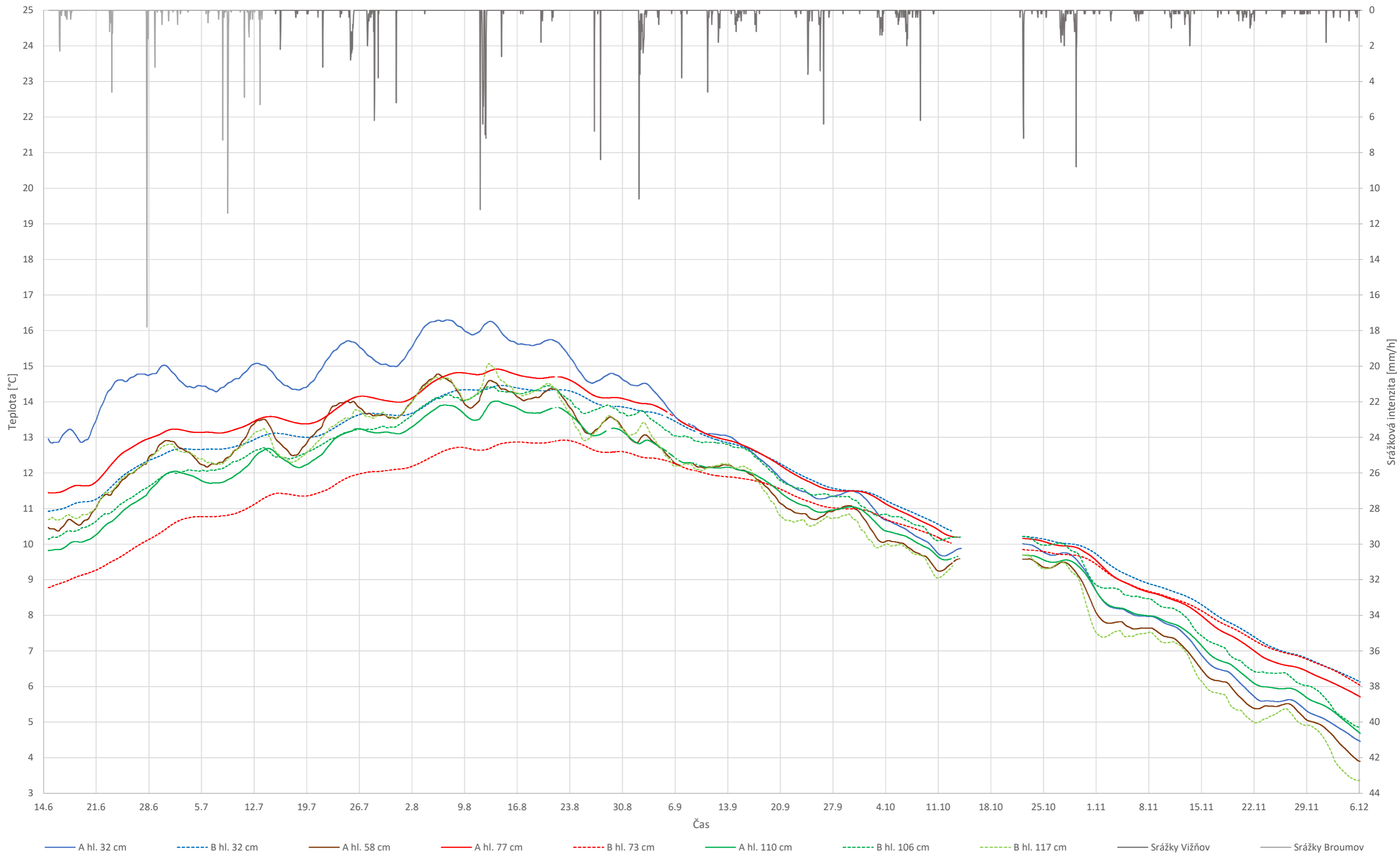
Příloha č. 6 - Teploty měřené tenzometry ve stanovištích A a B
