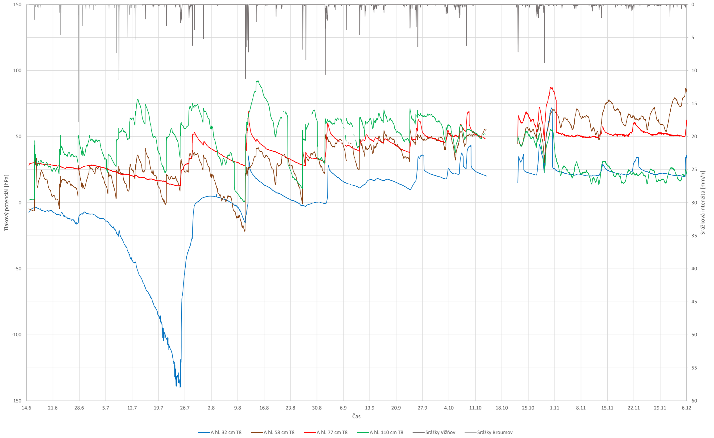
Příloha č. 2 - Tenzometry T8, stanoviště A
