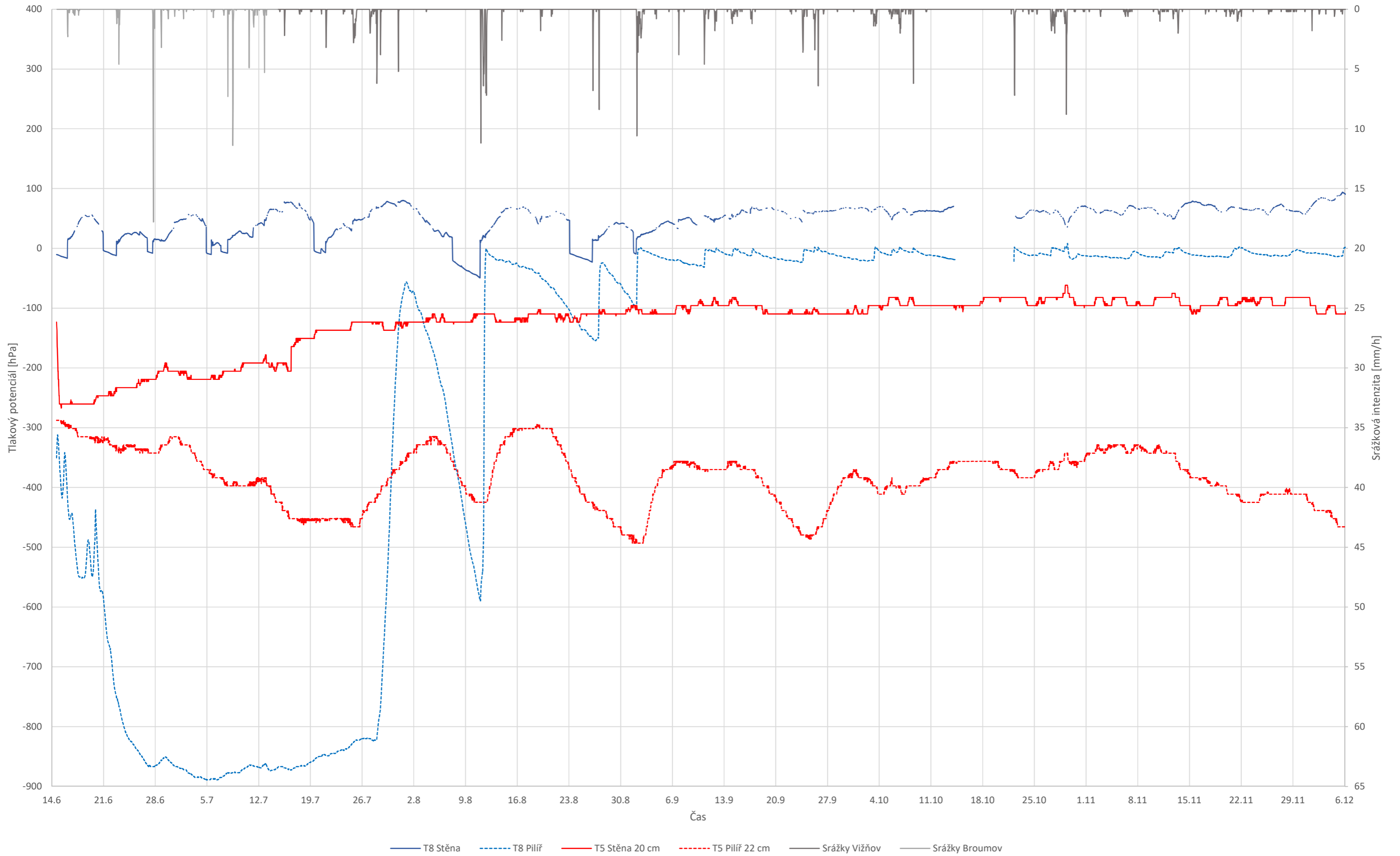
Příloha č. 4 - Tenzometry T5 a T8 instalované uvnitř kostela
