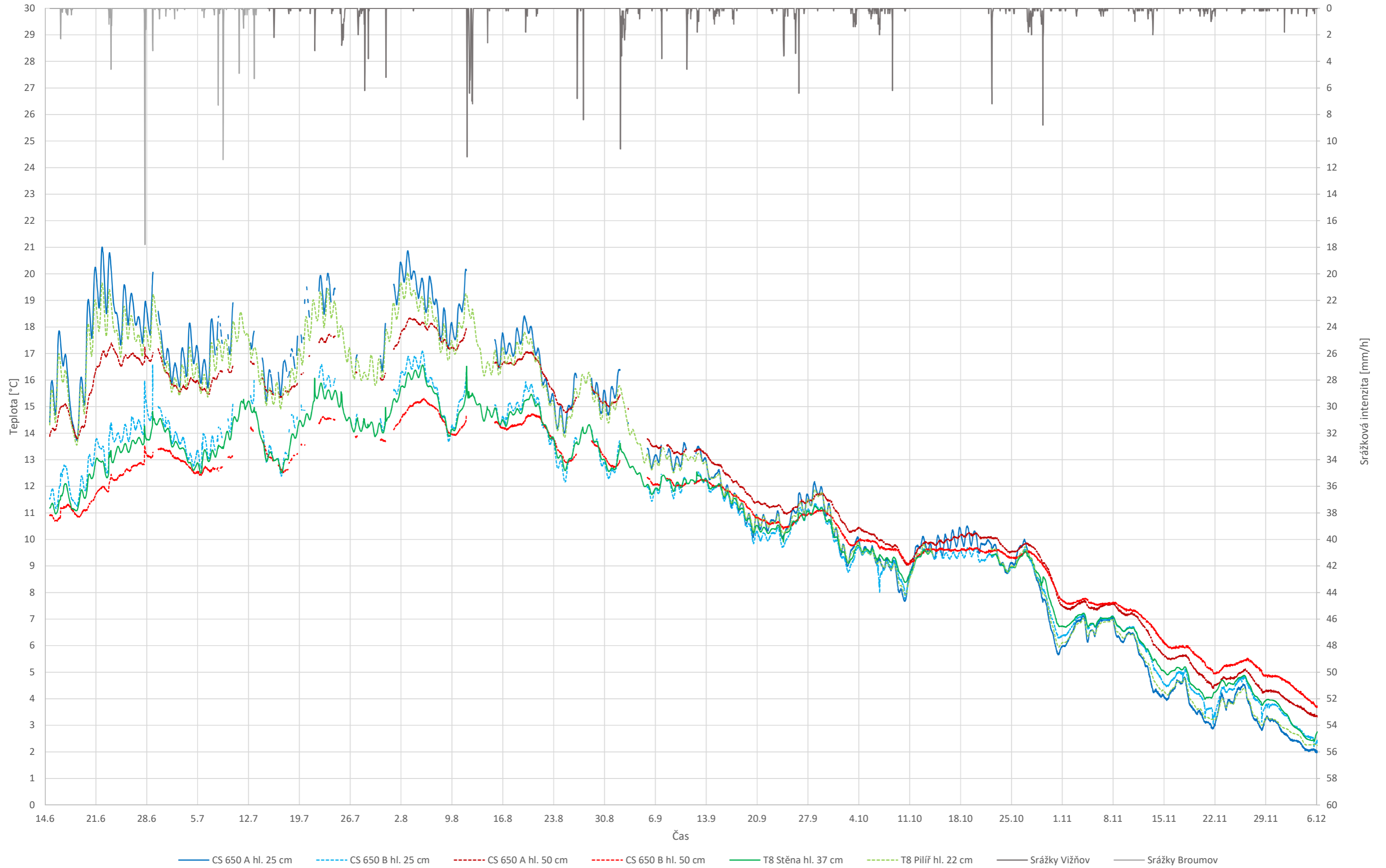
Příloha č. 7 - Porovnání teplot měřených vlhkostními čidly CS 650 a tenzometry T8 v kostele
