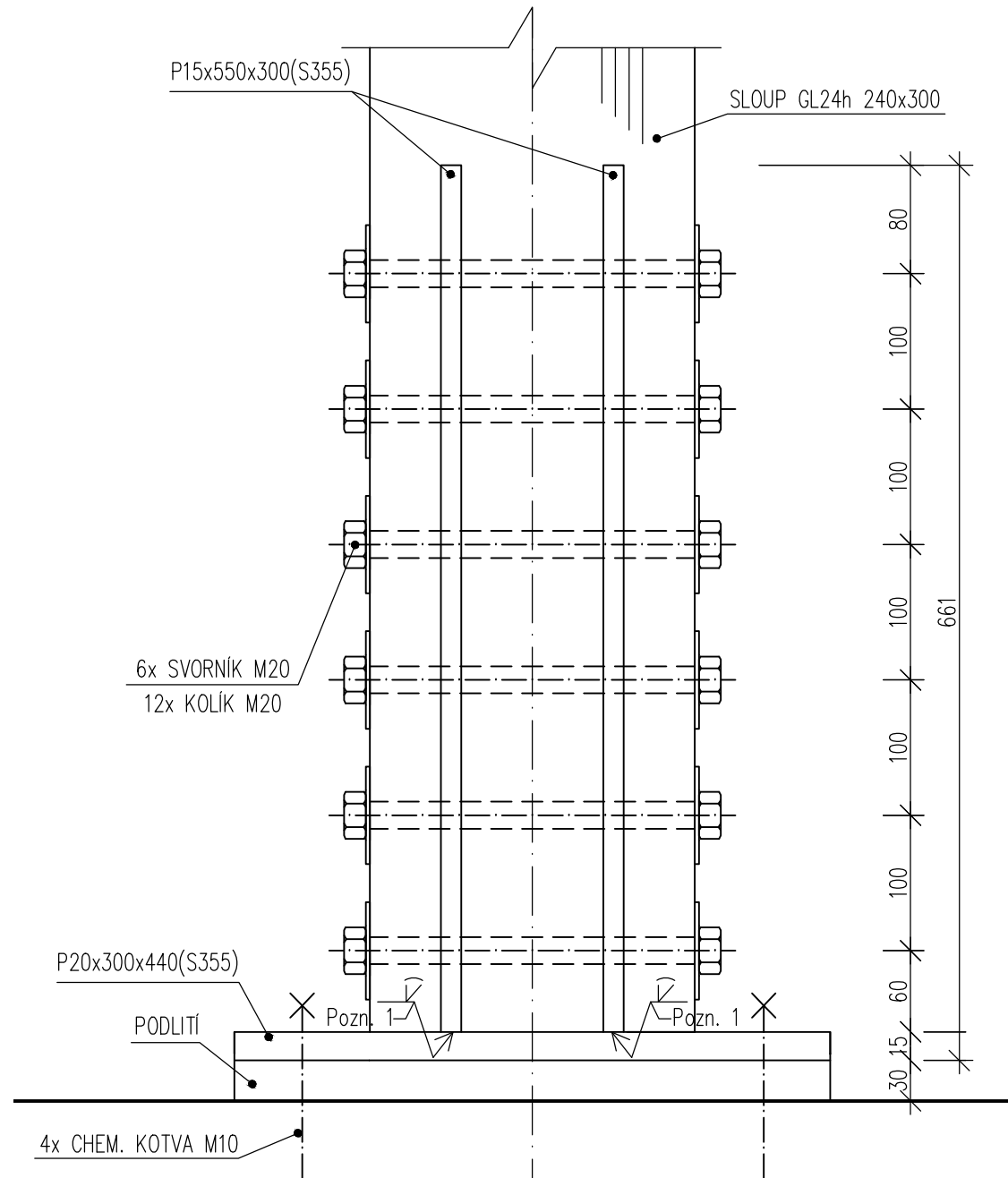
ŘEZ, M=1:5
