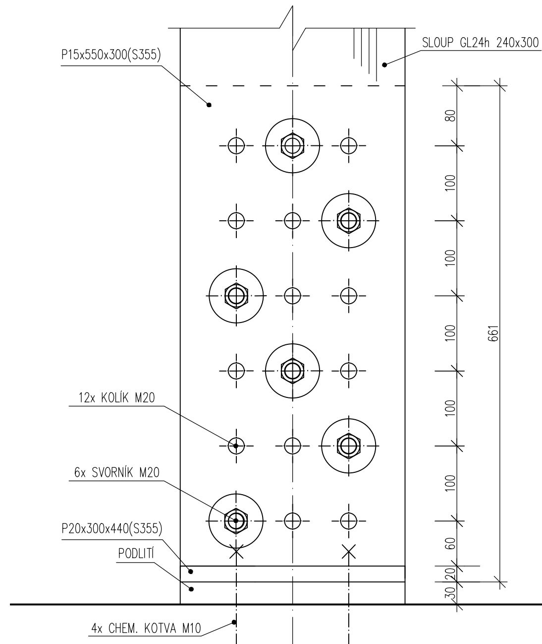
POHLED 2-2, M=1:5
