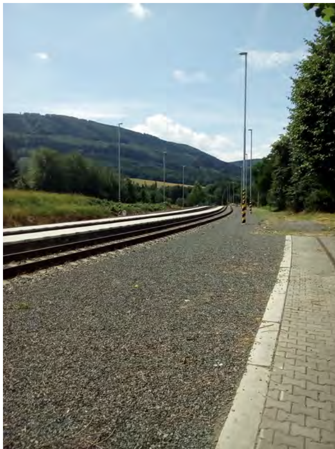
Foto 17: pohled na nástupiště v oblouku
