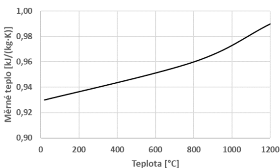
Graf 41 Měrné teplo – HB11
