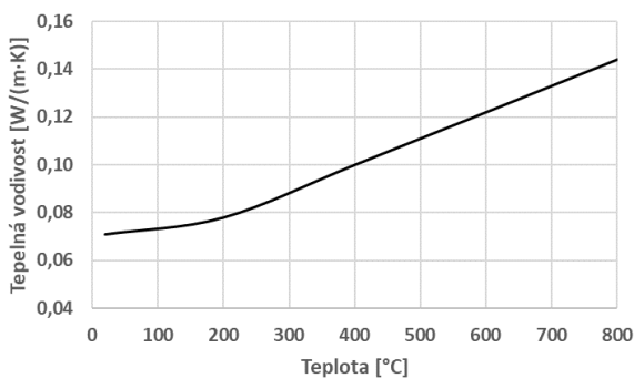
Graf 43 Teplená vodivost – Kerasil 1000
