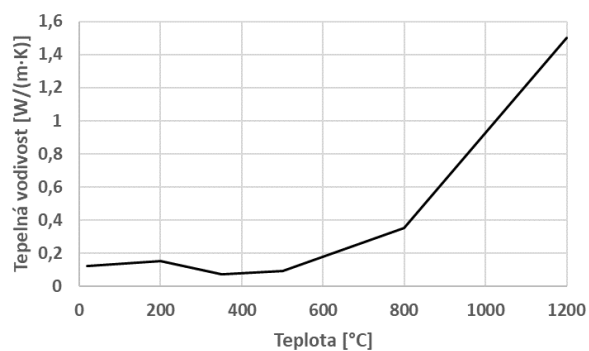
Graf 50 Teplená vodivost – Dřevo
