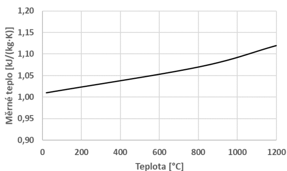
Graf 39 Měrné teplo – AT60A
