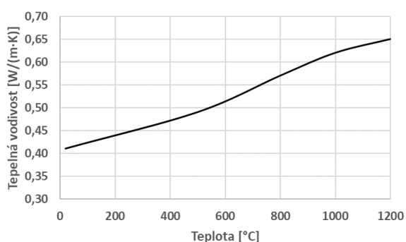
Graf 42 Teplená vodivost – HB11
