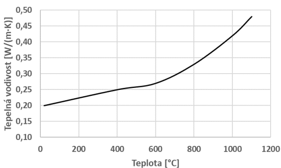
Graf 47 Teplená vodivost – Žárobeton
