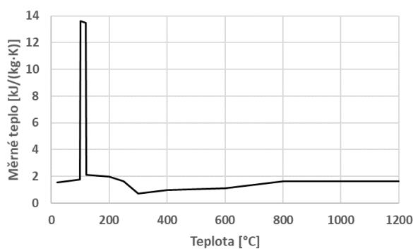
Graf 51 Měrné teplo – Dřevo
