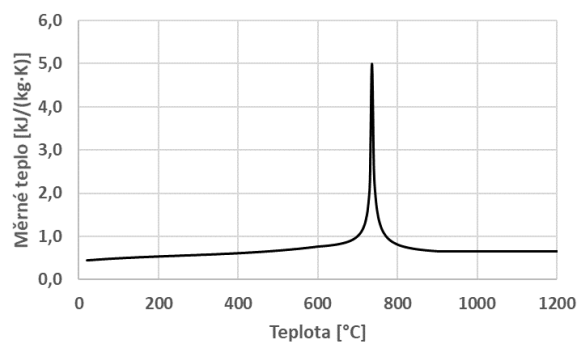
Graf 48 Měrné teplo – Ocel
