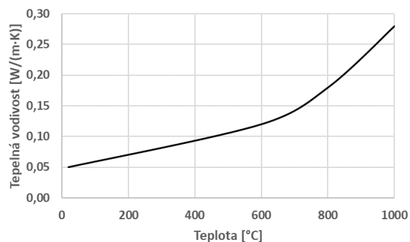
Graf 46 Teplená vodivost – Fibratec
