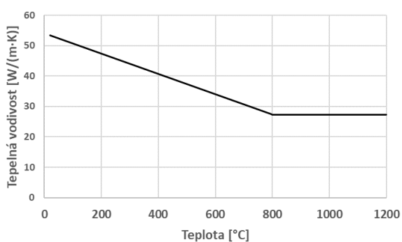
Graf 49 Teplená vodivost – Ocel
