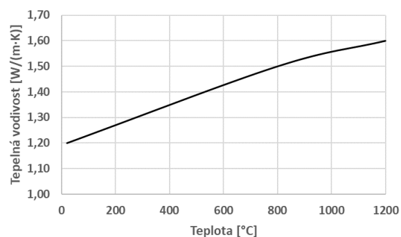
Graf 40 Teplená vodivost – AT60A
