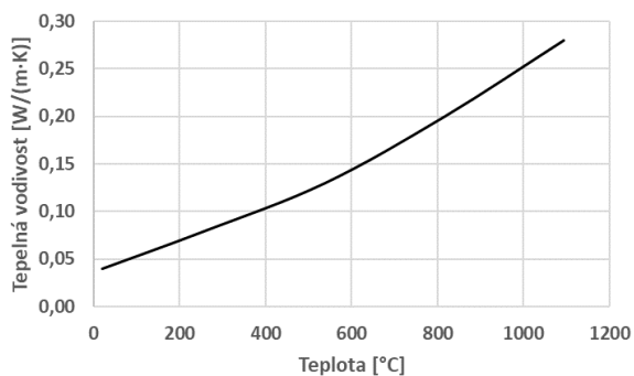
Graf 44 Teplená vodivost – Kerablok
