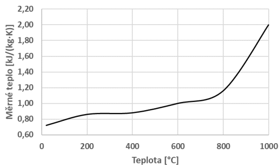
Graf 45 Měrné teplo – Fibratec
