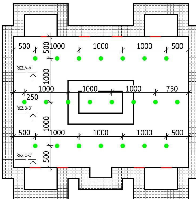
Obr. 46 Půdorys modelu
