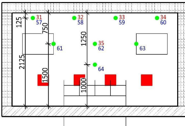
Obr. 49 Řez modelem C-C'
