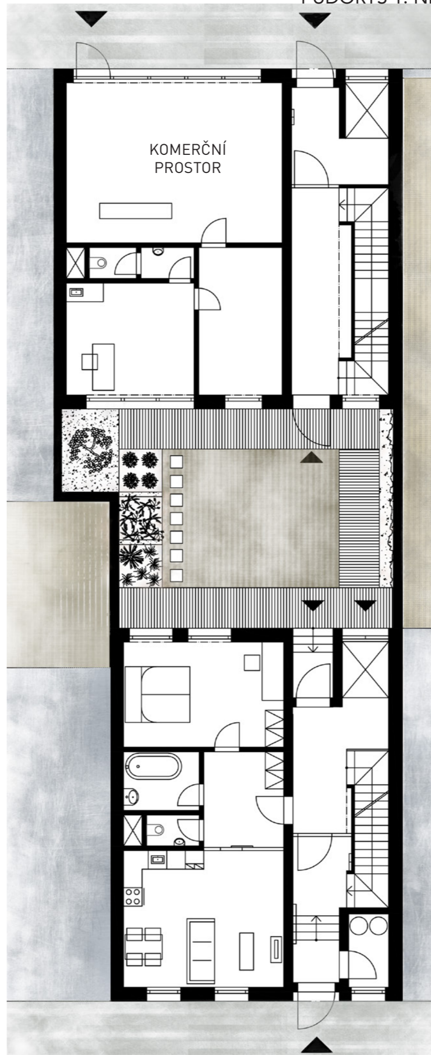
PŮDORYS 1. NP
