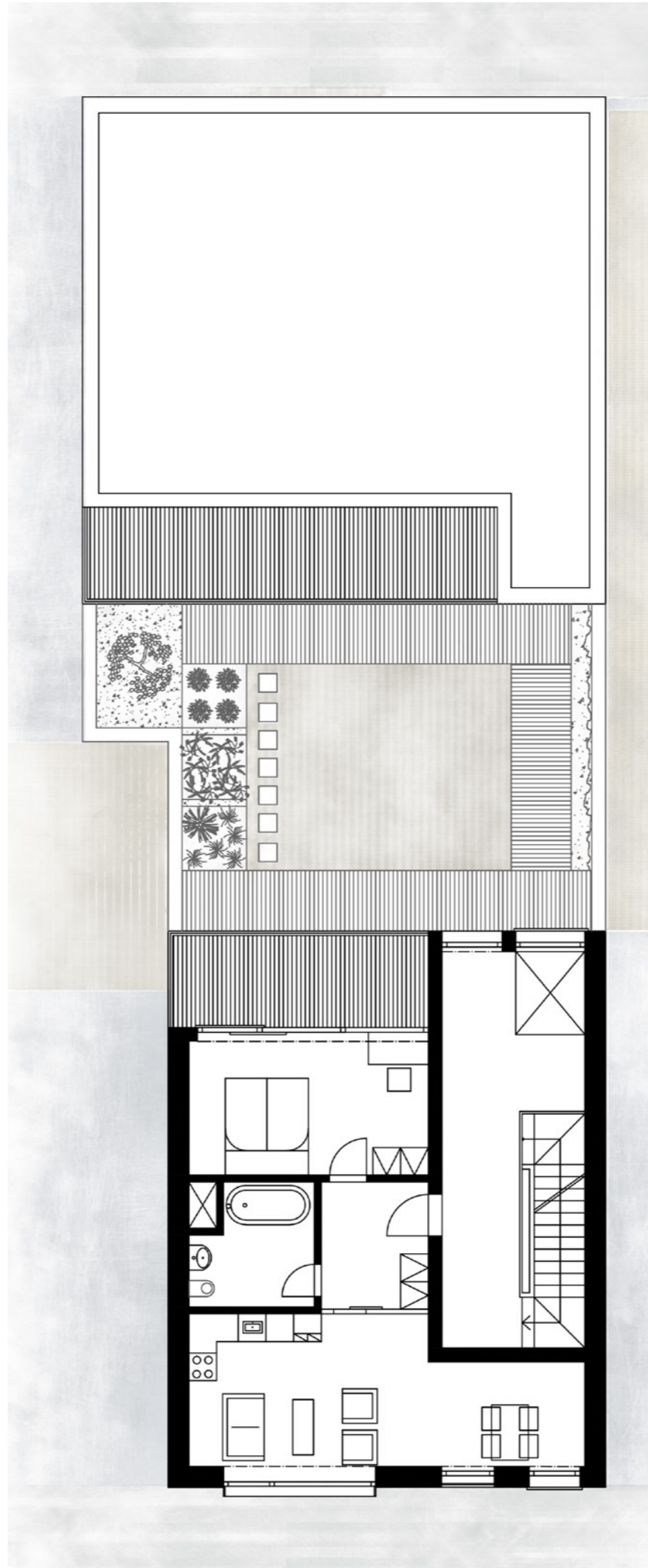
PŪDORYS 4. NP
