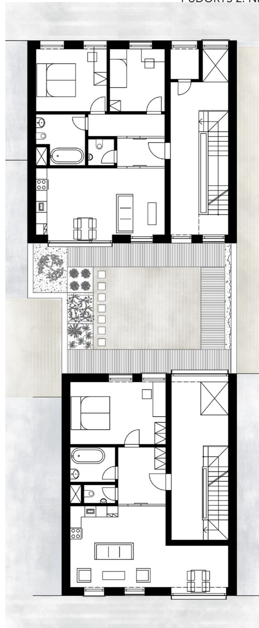
PŮDORYS 2. NP
