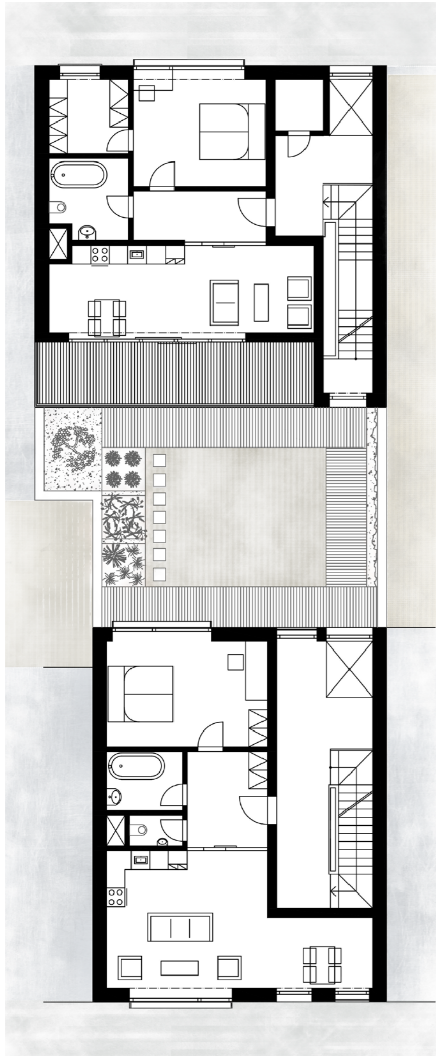
PŪDORYS 3. NP
