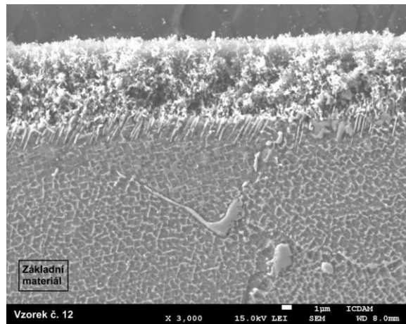
Alitační a difuzní vrstva
