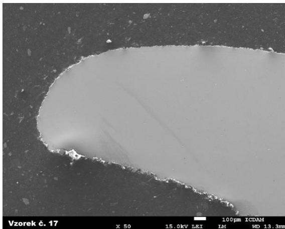
Náběžná hrana
