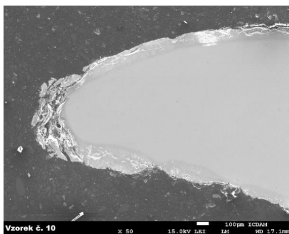
Alitační vrstva
