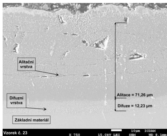
Alitační a difuzní vrstva
