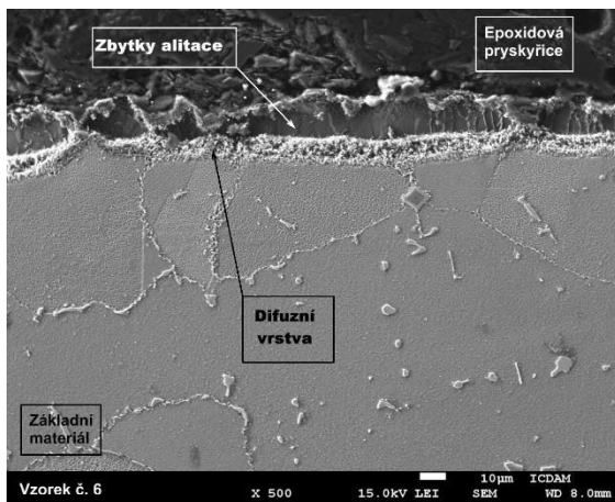
Alitační vrstva
