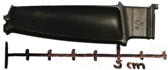
Hodnocená lopatka
