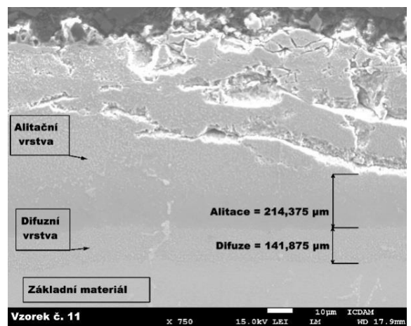
Alitační a difuzní vrstva
