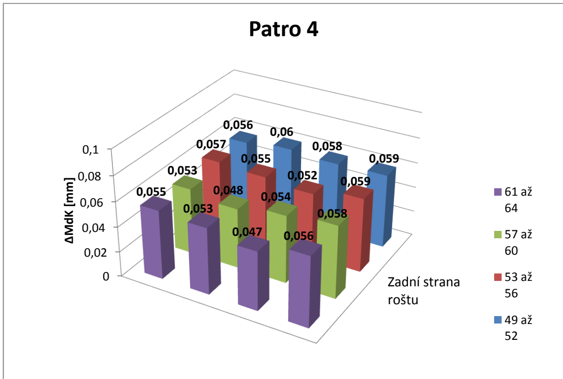
Příloha 9 : Vliv kalení na parametr Mdk – Patro 4
