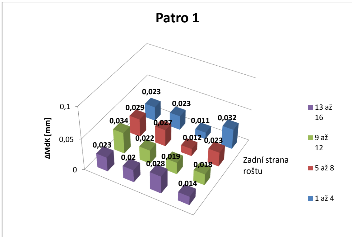
Příloha 9 : Vliv kalení na parametr MdK – Patro 1
