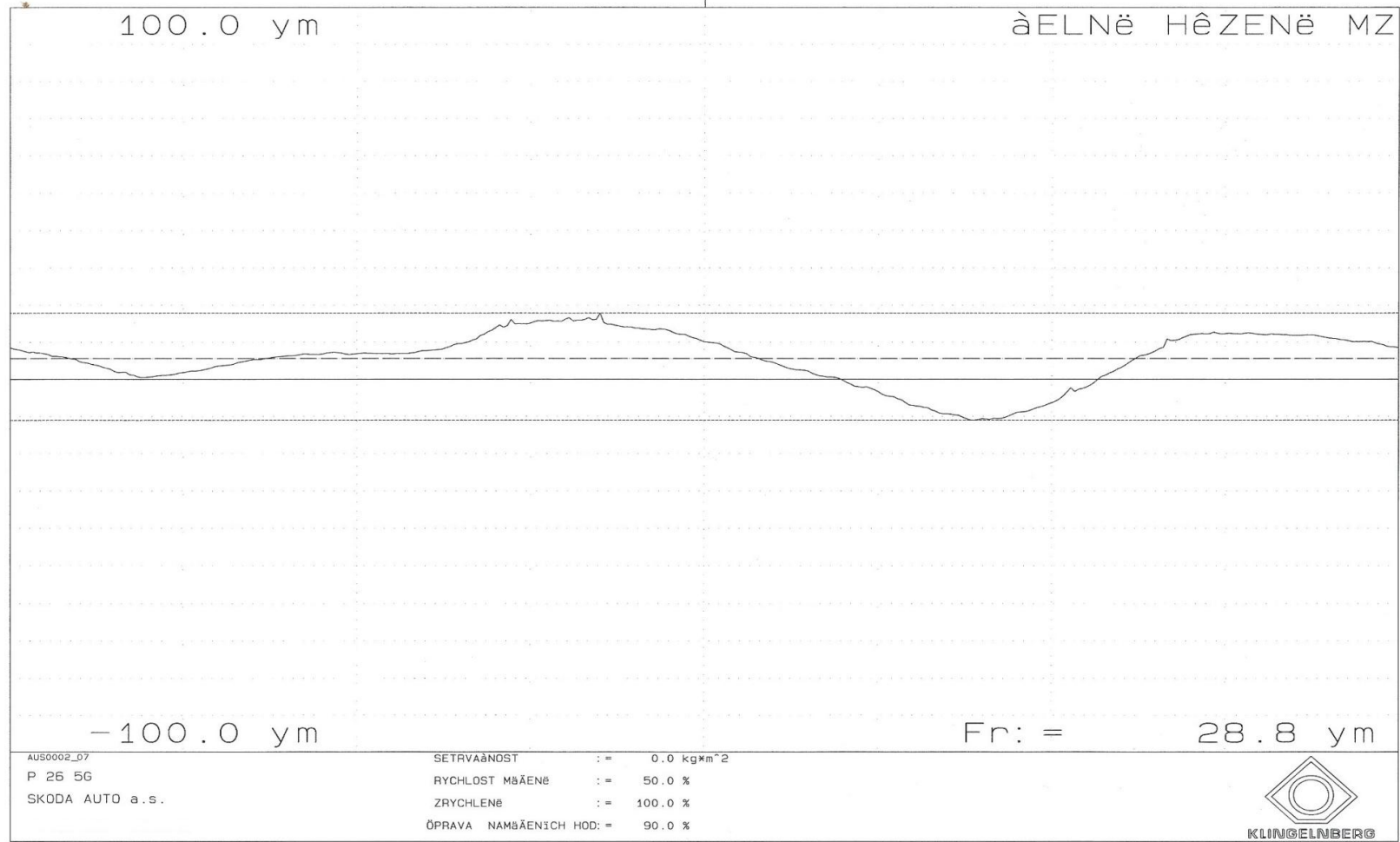
Přiloha 7: Protokol měření axiálního házení vñnce
