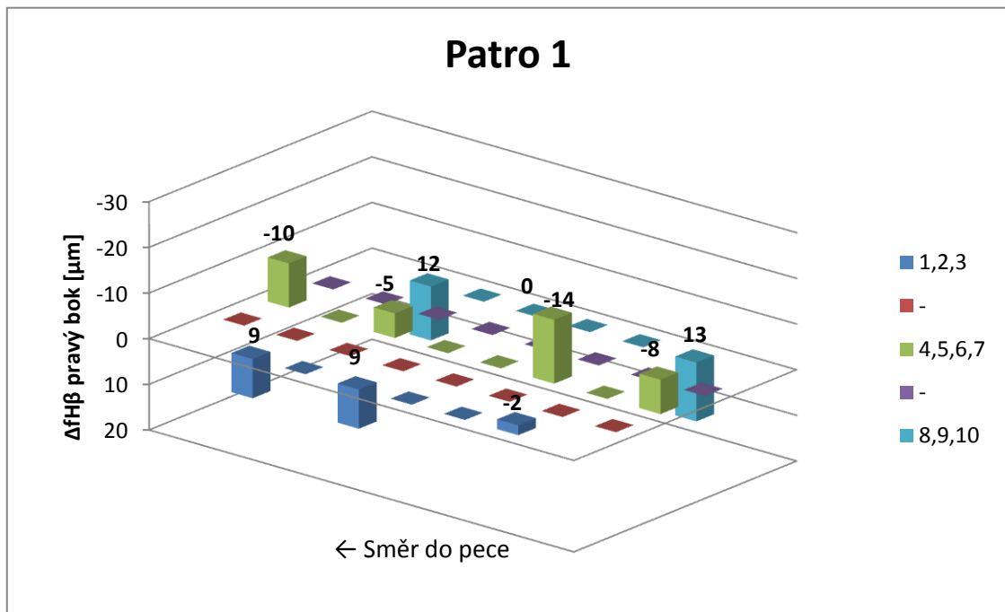
Příloha 10 : Vliv kalení v plynu na parametr fH \beta (pravý bok)-Patro 1
