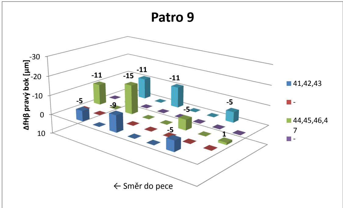
Příloha 10: Vliv kalení v plynu na parametr fHβ (pravá strana)-Patro 9
