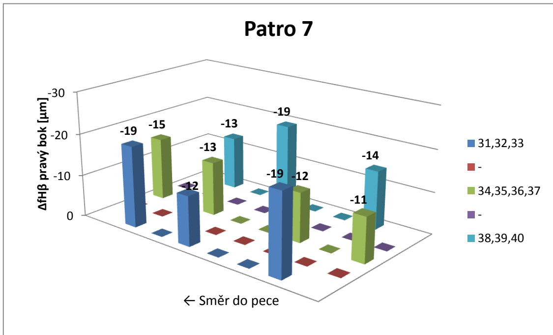
Příloha 10: Vliv kalení v plynu na parametr fHβ (pravý bok)-Patro 7
