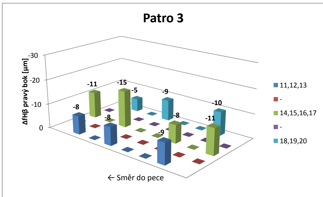
Příloha 10: Vliv kalení v plynu na parametr fH \beta (pravý bok)-Patro 3
