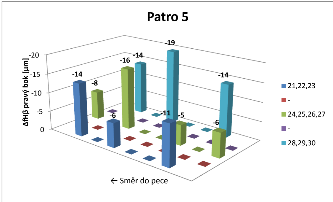
Příloha 10: Vliv kalení v plynu na parametr fHβ (pravý bok)-Patro 5
