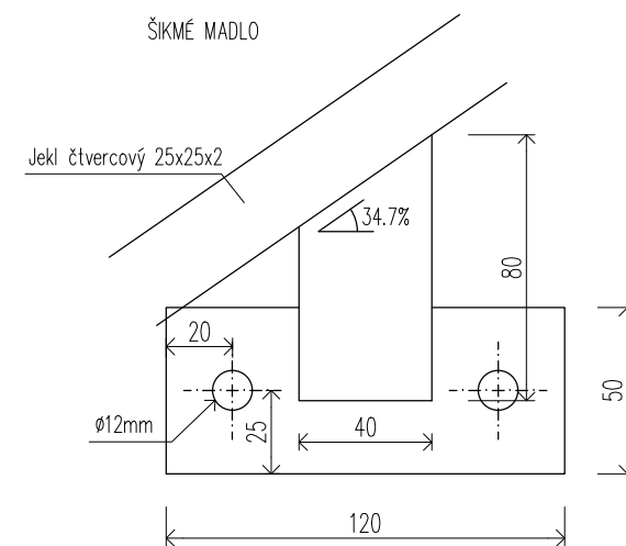
UCHYČENÍ MADLA – ČELNÍ POHLED
