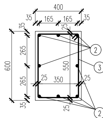
ŘEZ A-A'
