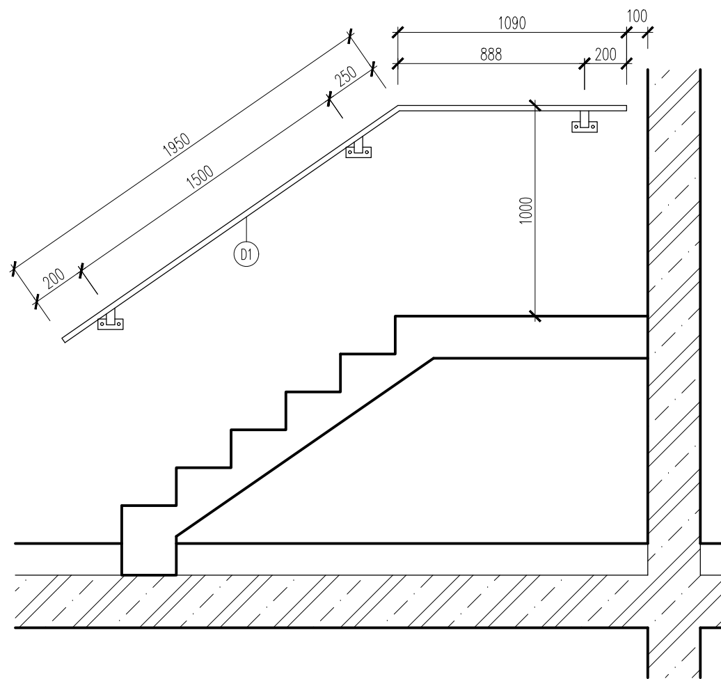
UCHYČENÍ MADLA – ČELNÍ POHLED
