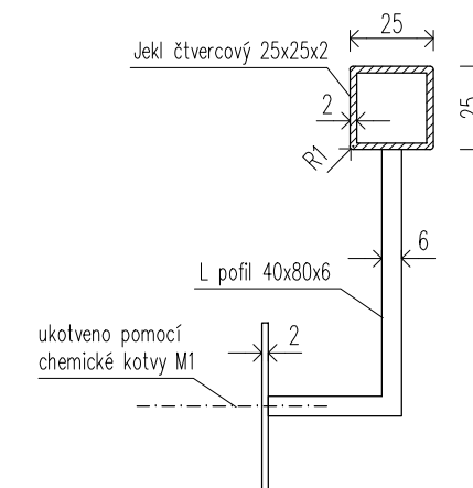
UCHYČENÍ MADLA – BOČNÍ POHLED
