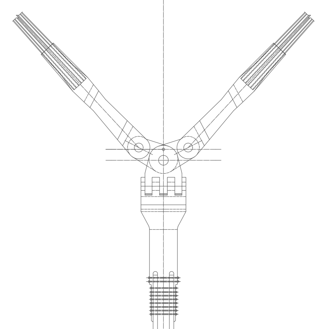
DETAIL KOTVENÍ TÁHLA
