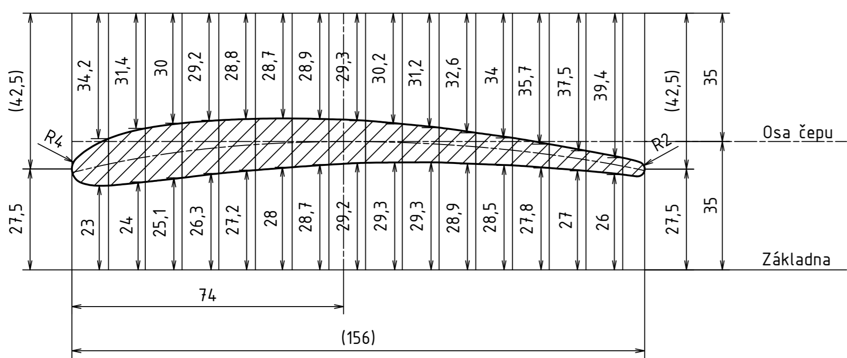
TVAR PROFILU ROZVÁDĚČÍ LOPATKY
