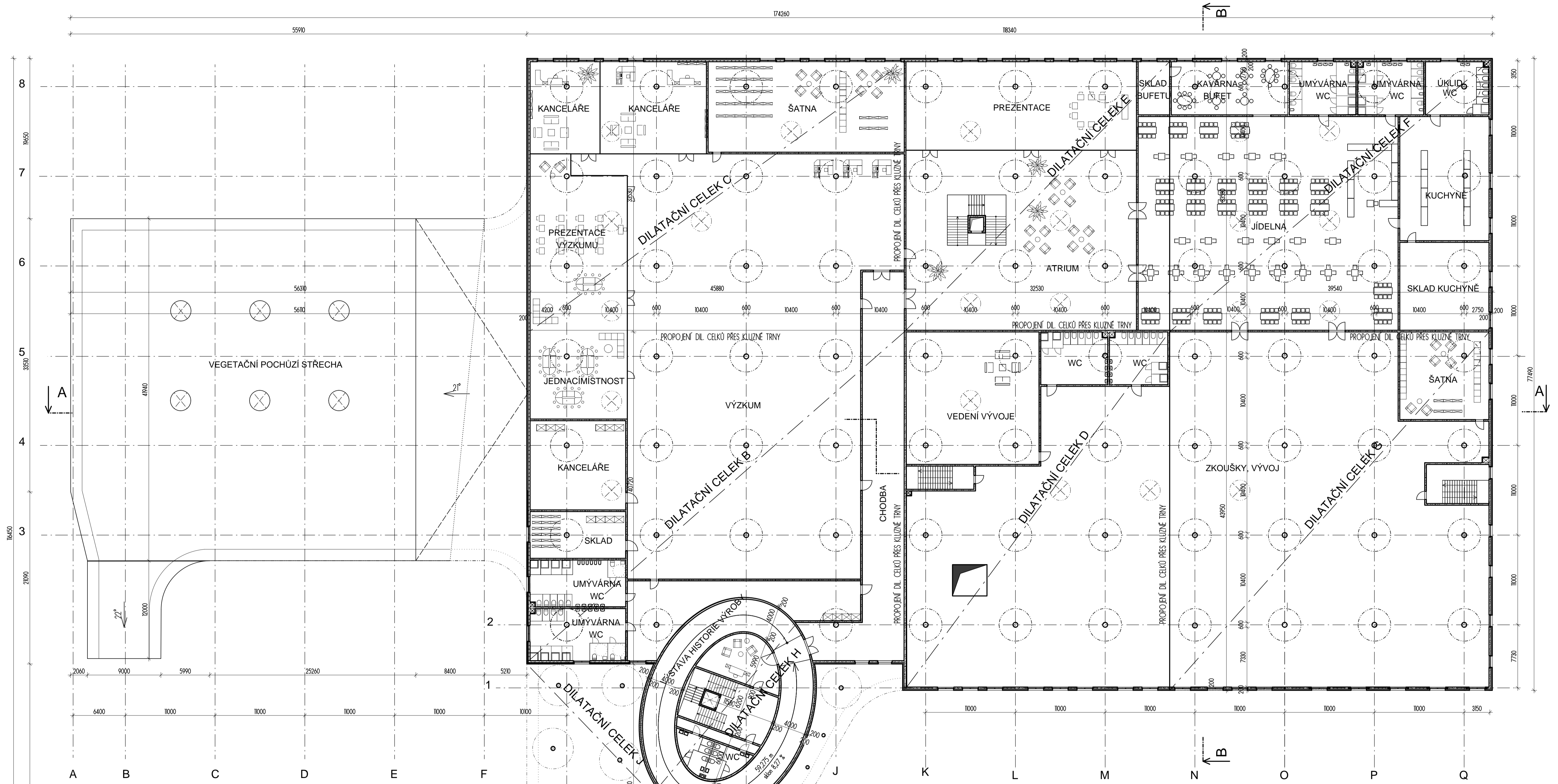
SCHÉMATICKÝ PŮDORYS 3-6.NP - STUDIE M 1:250
