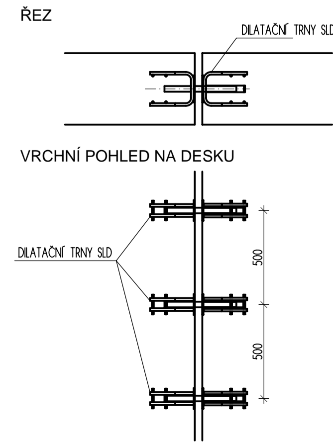
SCHÉMA NAPOJENÍ DESEK DILATAČNÍCH CELKŮ M1:20
