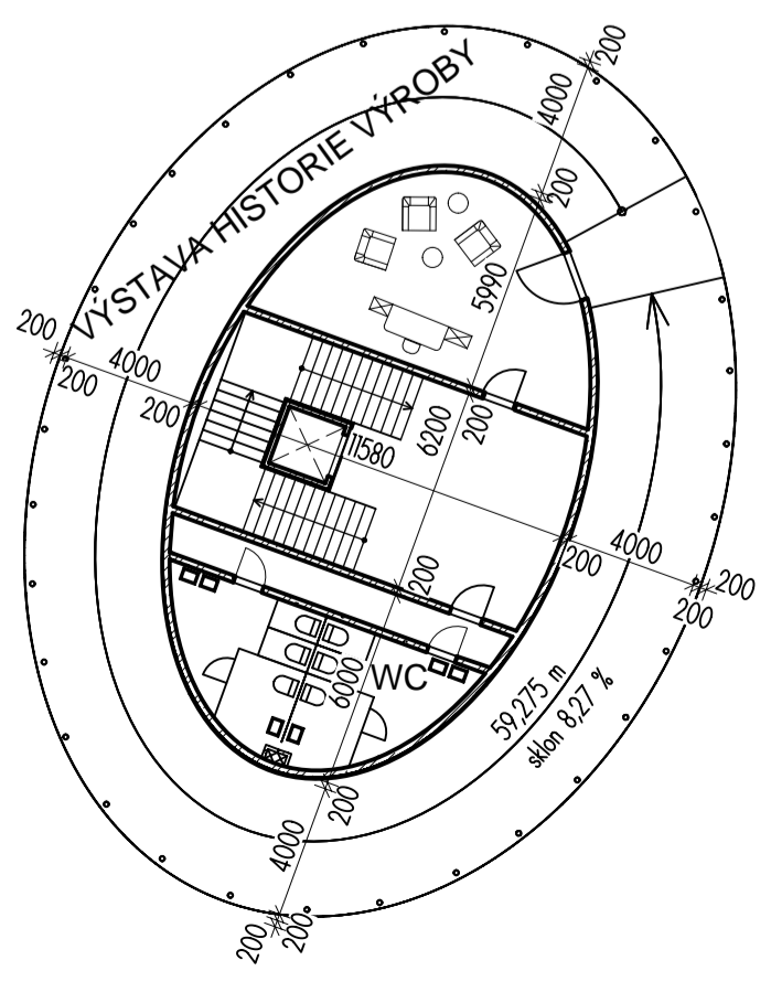
SCHÉMATICKÝ PŮDORYS 3-6.NP - STUDIE M 1:250
