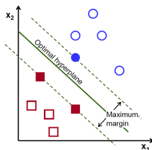
Obrázek 3.2. Ukázka použití metody SVM [29].
