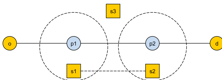
Obrázek 4.2. Princip hledání možných zastávek na trase mezi body o a d . Zastávky s1 a s2 leží v blízkosti bodů p1 a p2 , na kterých došlo ke změně dopravního módu - proto jsou přidány do množiny C .
