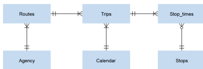
Obrázek 4.1. Entity-Relationship diagram povinných souborů GTFS balíčku.
