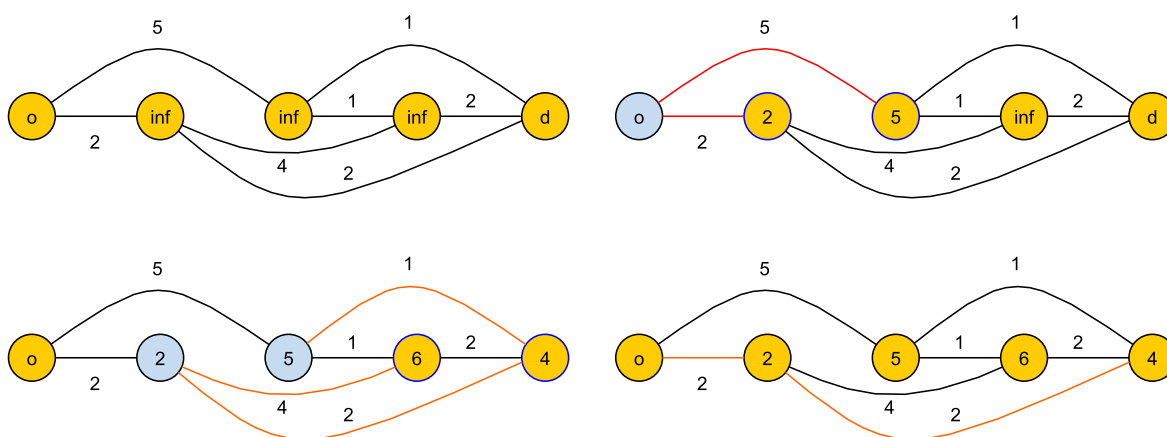
Obrázek 4.4. Ukázka algoritmu pro hledání nejkratší cesty mezi body o a d , na posledním obrázku je pak znázorněn i její průběh. V první fázi nastavíme ohodnocení všech uzlů na hodnotu inf a algoritmus začneme v takovém uzlu, která obsahuje pouze výstupní a žádnou vstupní hranu. V každé další iteraci je aktualizována hodnota uzlu s ohledem na její minimalizaci. Uzel je uzavřen v momentě, kdy začneme zpracovávat jeho potomky, neboť díky topologickému uspořádání a acykličnosti se již nemůžeme vrátit.
