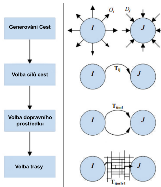
Obrázek 2.2. Schéma čtyřfázového modelu [9]. Nejprve nalezneme množiny vstupních a výstupních uzlů ( O a D ). Poté jednotlivé uzly spojíme trasou T_{ij} za využití prostředku m_1 a trasy r_1 .
