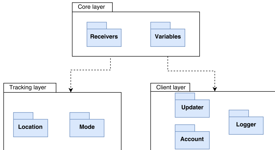
Obrázek 5.1. Diagram balíčků a jejich rozdělení do jednotlivých vrstev aplikace.
