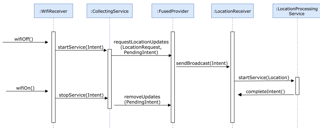
Obrázek 5.2. Diagram procesu zaznamenávání pozice.
