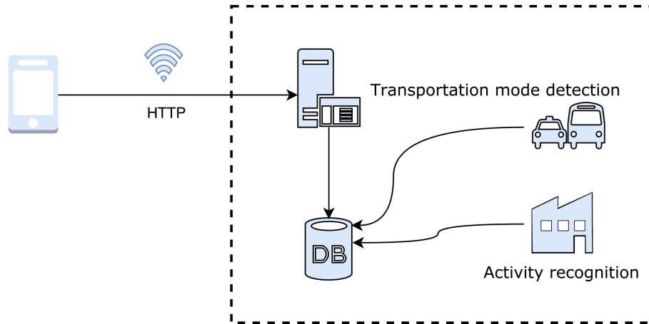
Obrázek 4.5. Návrh architektury systému pro aktivně-cestovní průzkum.
