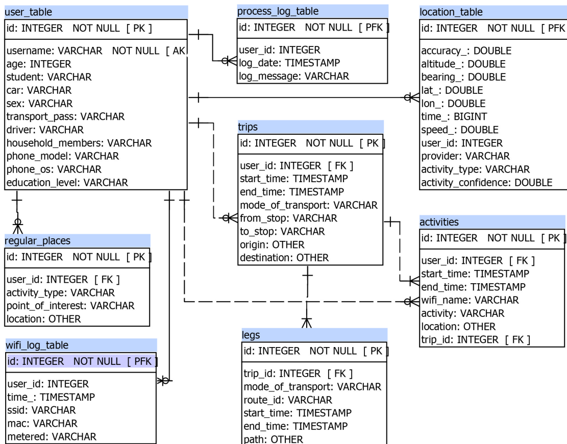
Obrázek 6.1. Databázové schéma všech tabulek systému pro aktivně-cestovní průzkum.
