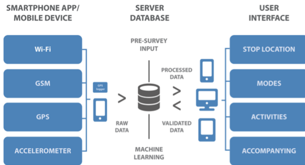
Obrázek 3.1. Schéma architektury systému FMS. Zdroj: https://its.mit.edu/future-mobility-sensing .
