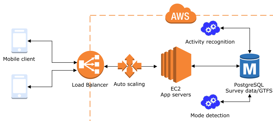
Obrázek 6.2. Architektura poskytovaného systému.
