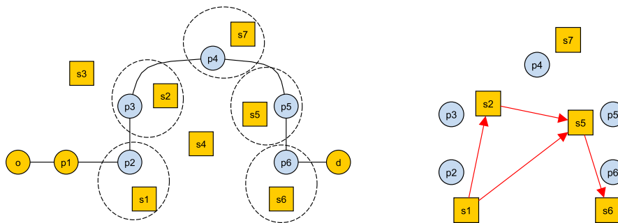
Obrázek 4.3. Konstrukce grafu G . Modře znázorněné body odpovídají souřadnicím, kde došlo ke změně dopravního módu a zároveň je v jejich blízkosti detekována zastávka MHD. Zastávky s_1, s_2, s_5 a s_6 jsou přidány do grafu G , zastávka s_7 je vyřazena z důvodu neexistujícího spojení s grafem.
