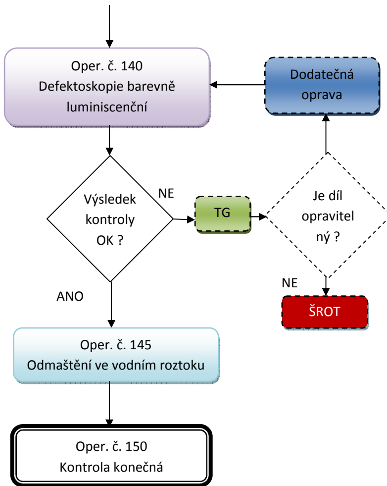
Obrázek 1: Procesní mapa výroby ochranného krytu
