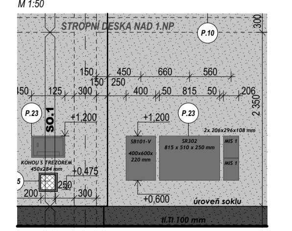
SCHEMA UMÍSTĚNÍ EL SKŘÍNÍ na FASÁDĚ M.1.01
