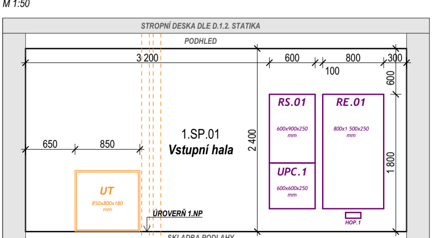
SCHEMA SESTAVY ROZVADĚČŮ M.1.02
